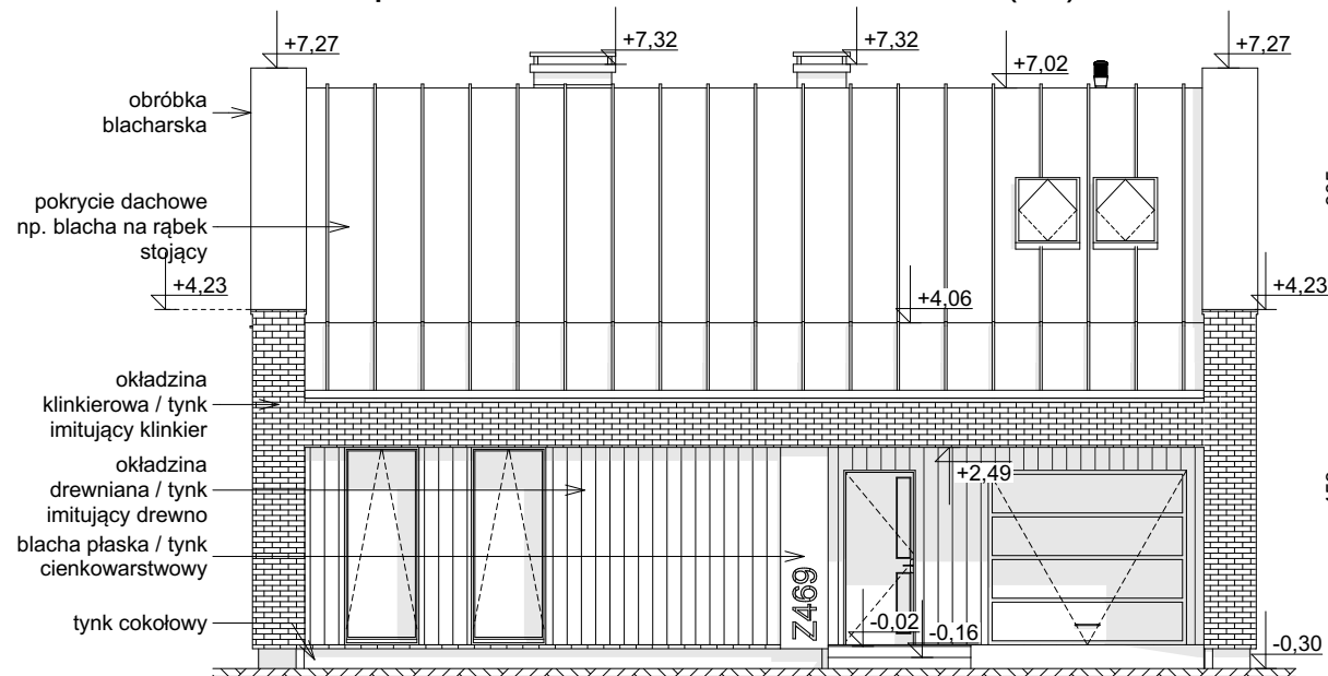
ELEVACJA FRONTOWA
