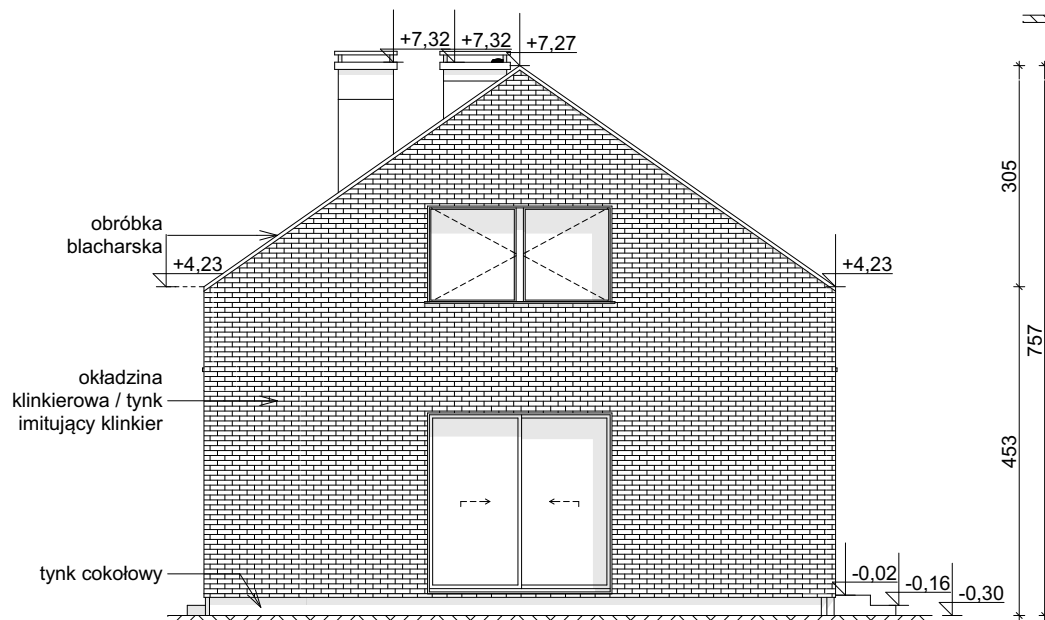
ELEVACJA BOCZNA
