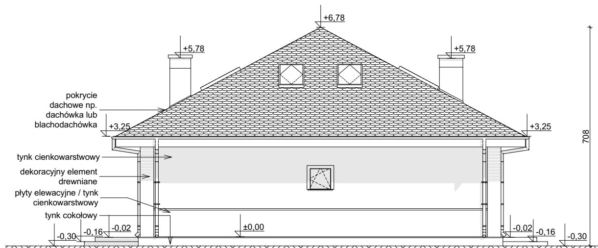
ELEWACJA BOCZNA
