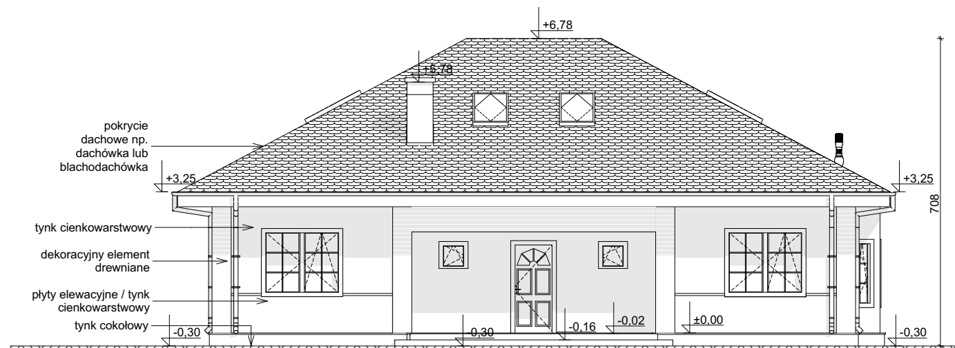
ELEWACJA FRONTOWA
