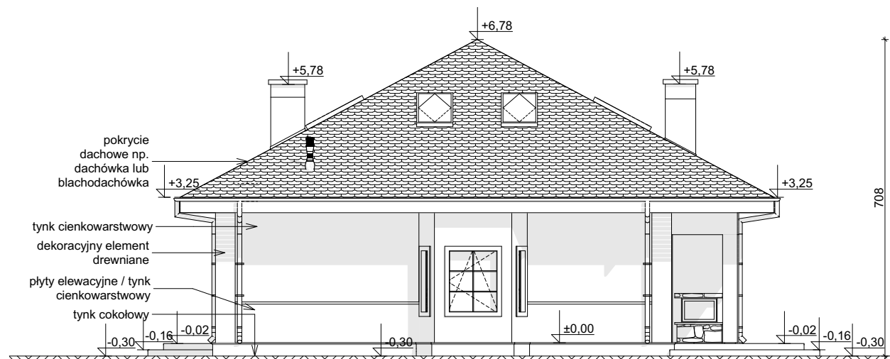
ELEWACJA BOCZNA
