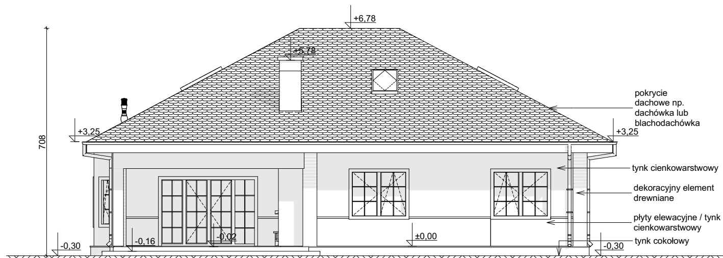
ELEWACJA OGRODOWA
