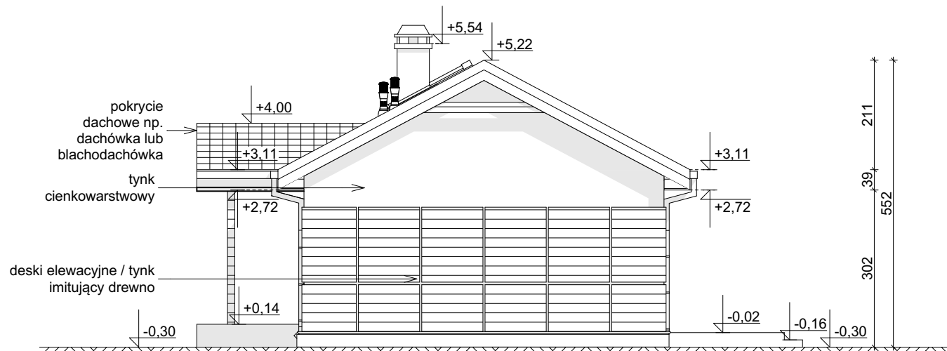
ELEWACJA BOCZNA
