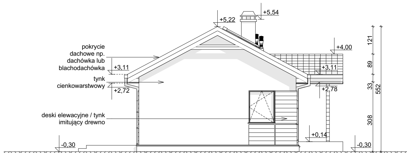
ELEWACJA BOCZNA
