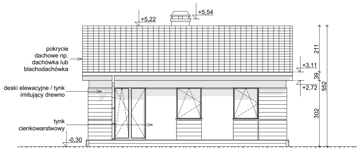
ELEWACJA OGRODOWA
