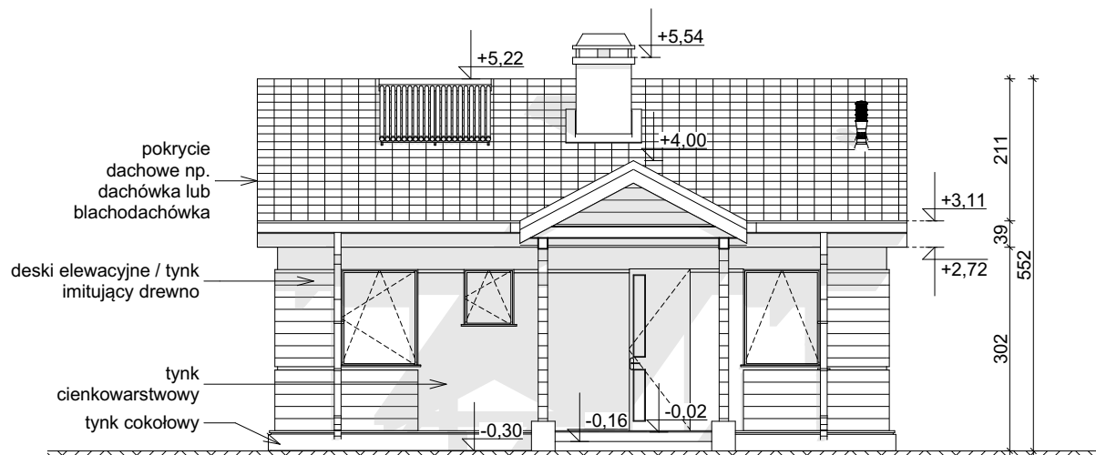
ELEWACJA FRONTOWA
