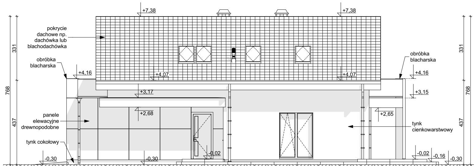
ELEWACJA FRONTOWA
