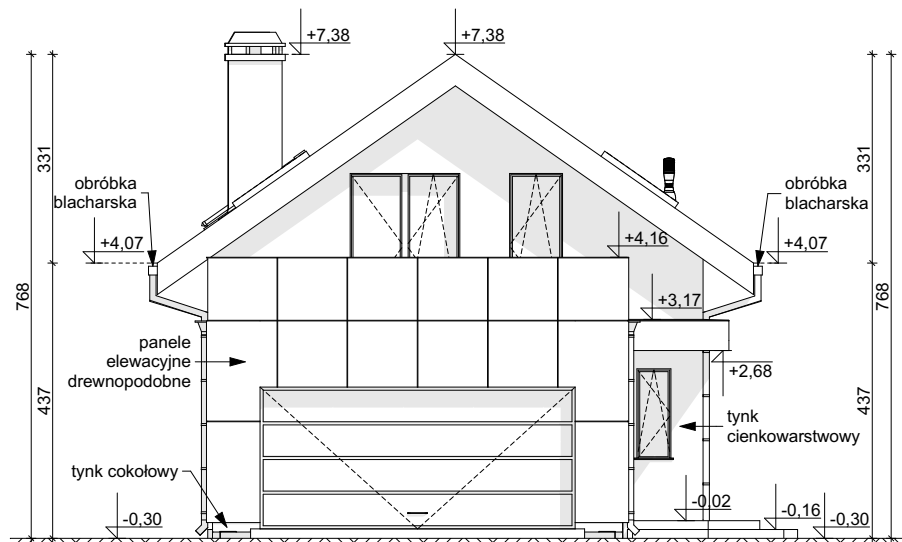
ELEWACJA BOCZNA
