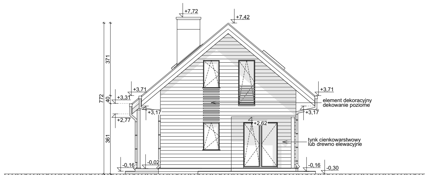
ELEVACJA BOCZNA
