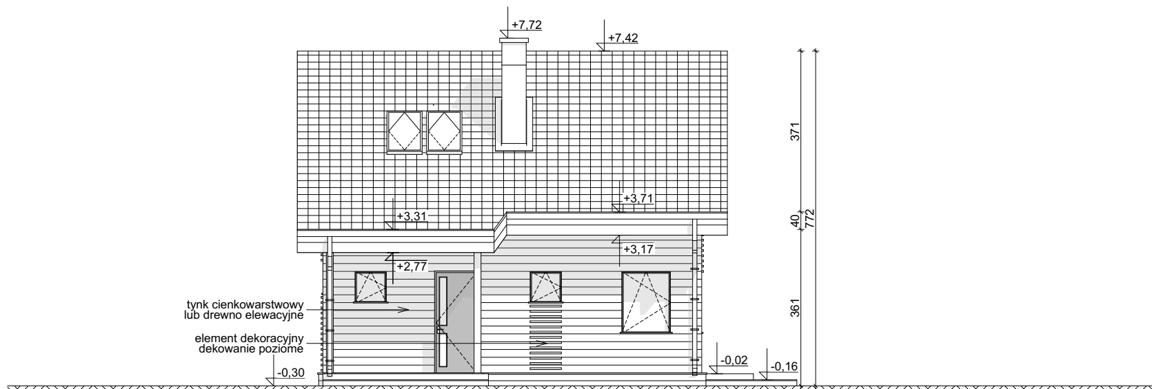
ELEWACJA FRONTOWA
