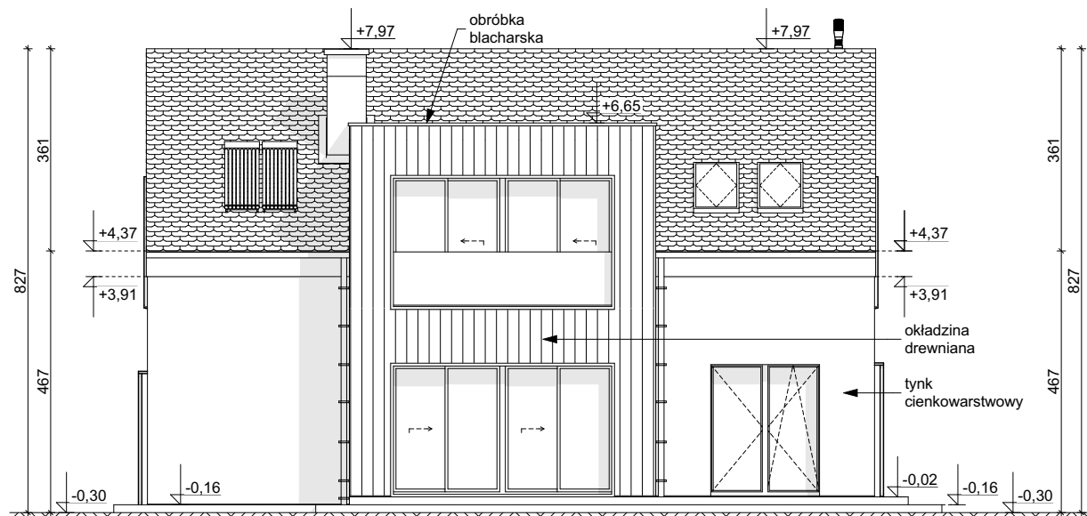
ELEWACJA OGRODOWA
