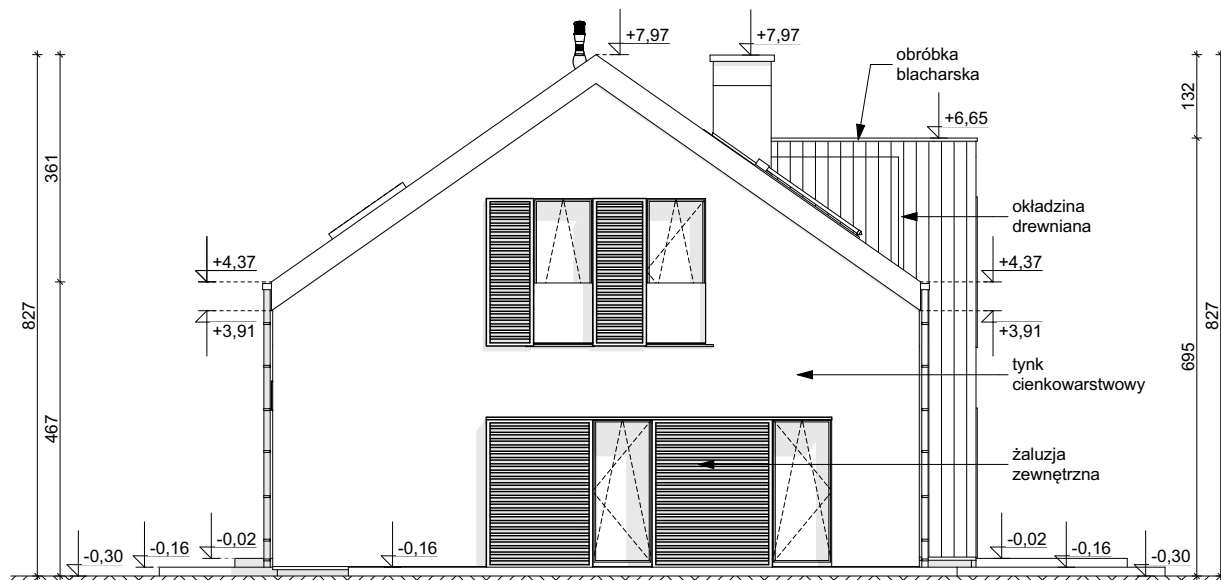
ELEWACJA BOCZNA
