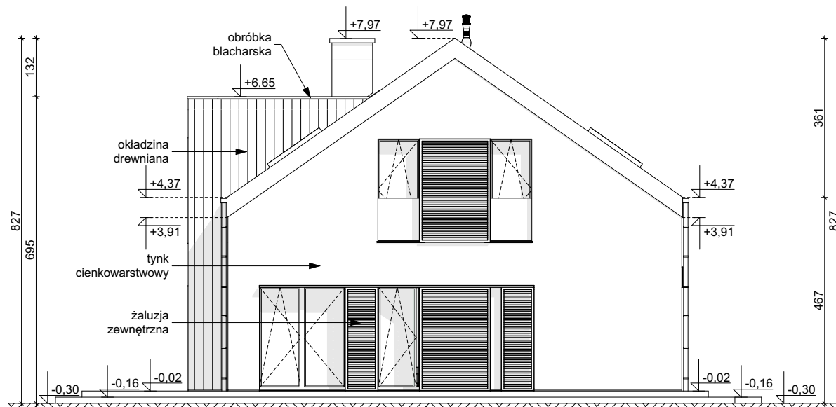
ELEWACJA BOCZNA
