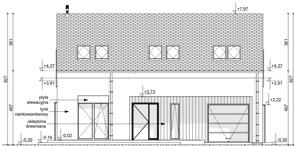
ELEWACJA FRONTOWA
