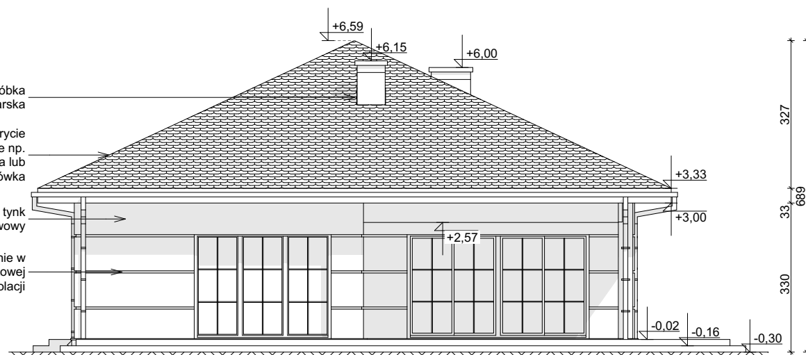
ELEWACJA OGRODOWA
