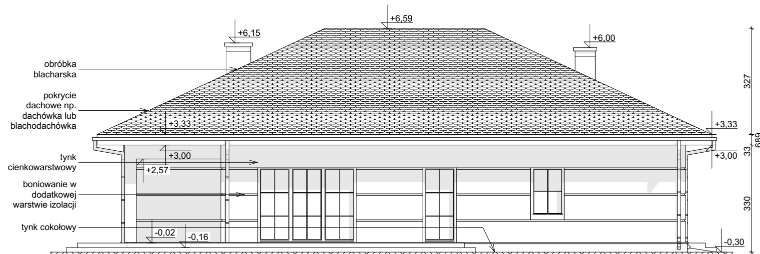
ELEWACJA BOCZNA
