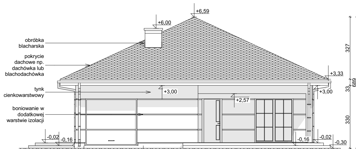
ELEWACJA FRONTOWA
