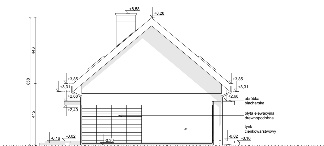
ELEWACJA BOCZNA
