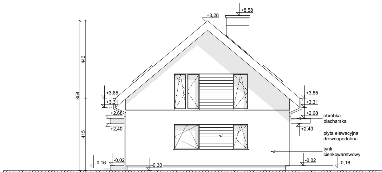
ELEWACJA BOCZNA
