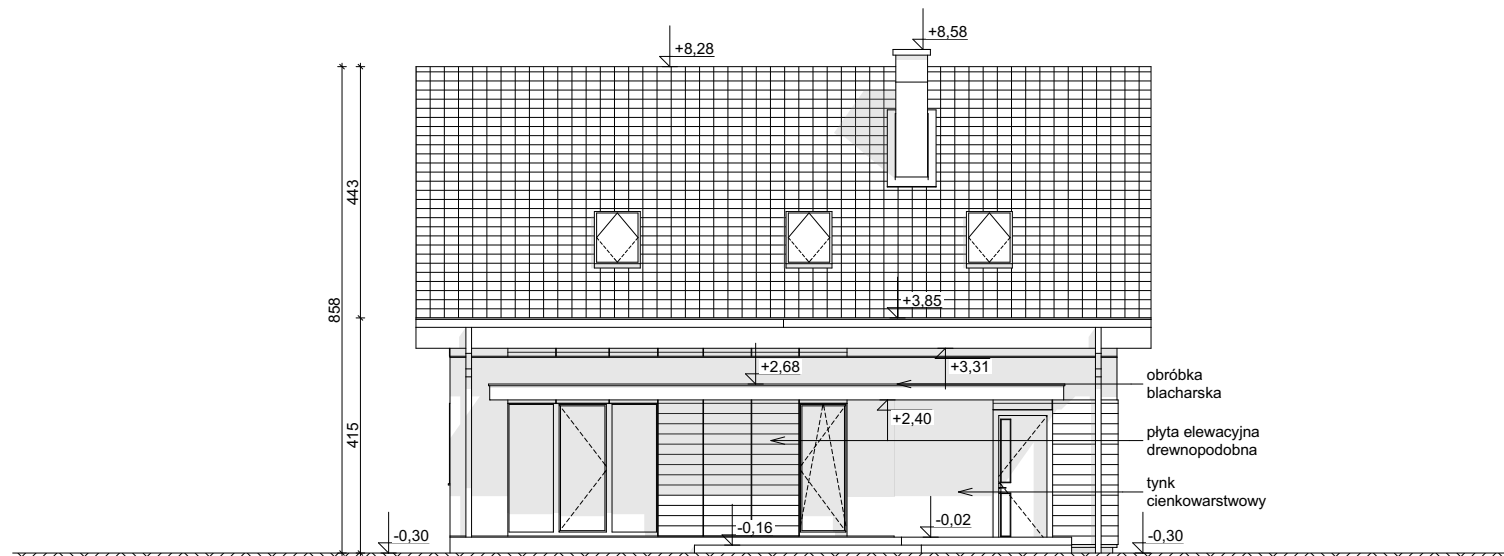
ELEWACJA OGRODOWA
