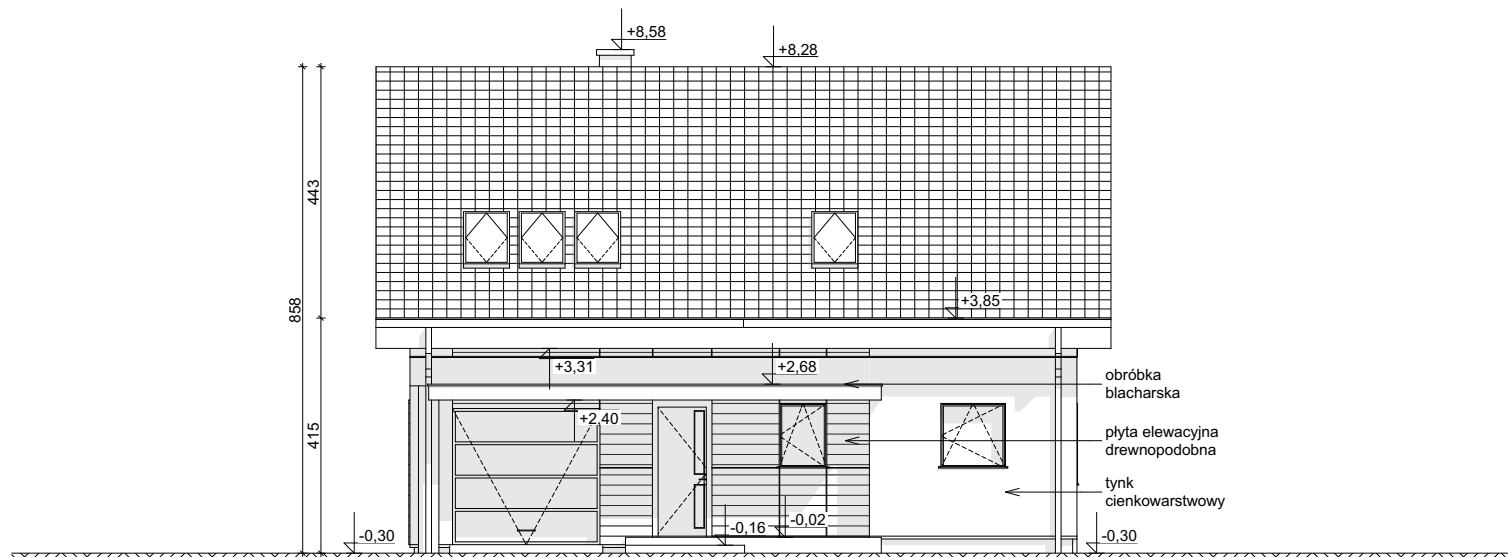
ELEWACJA FRONTOWA
