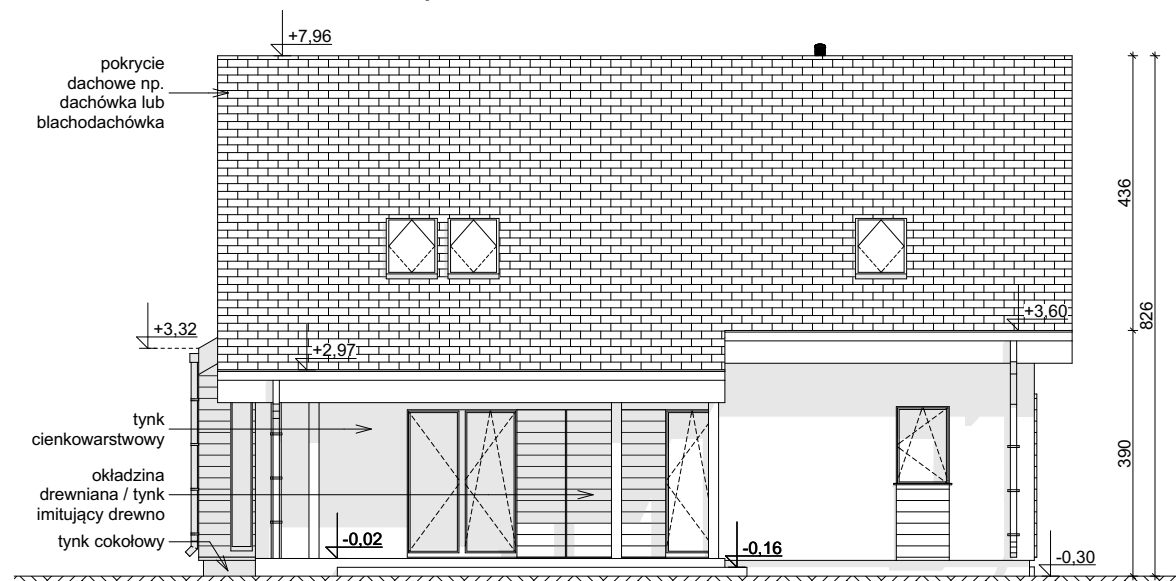
ELEWACJA OGRODOWA
