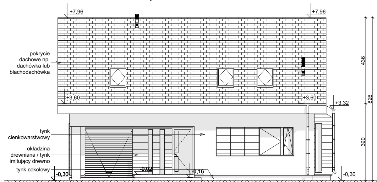
ELEWACJA FRONTOWA
