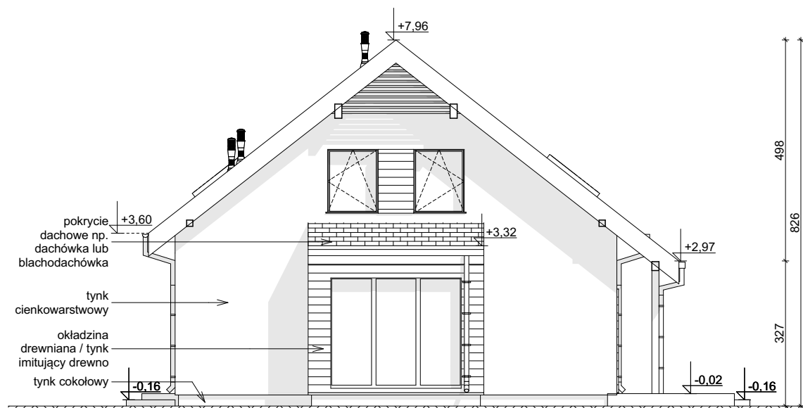
ELEWACJA BOCZNA
