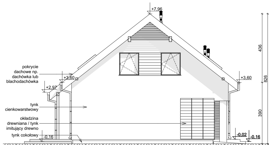
ELEWACJA BOCZNA
