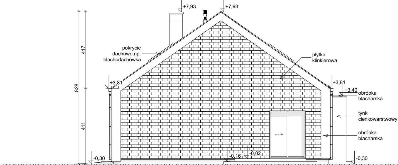
ELEWACJA BOCZNA
