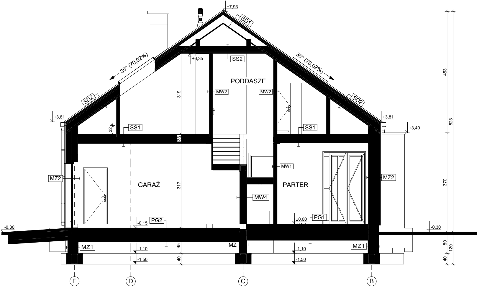
PRZEKRÓJ B-B
