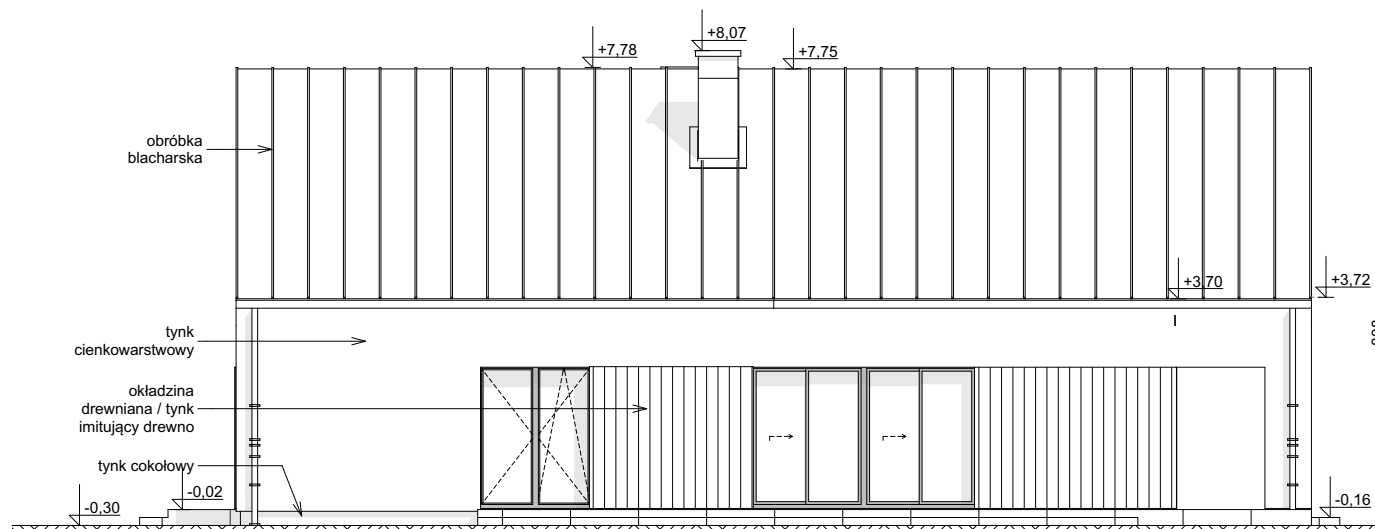
ELEWACJA BOCZNA
