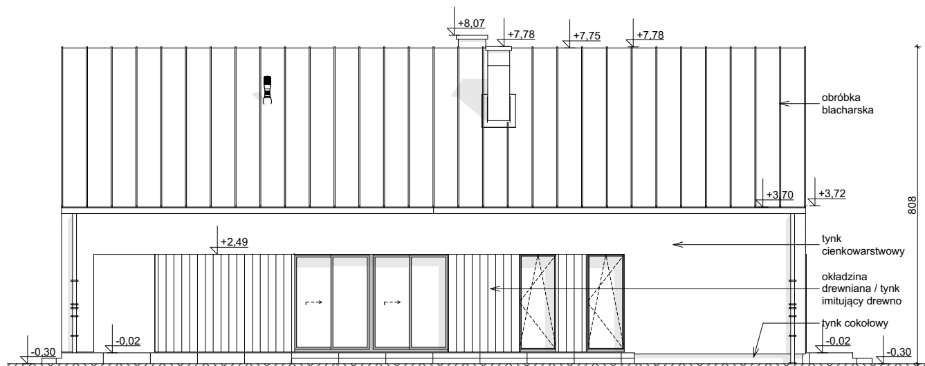
ELEWACJA BOCZNA
