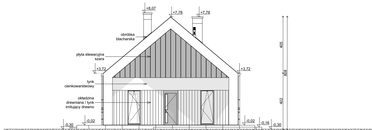
ELEWACJA FRONTOWA
