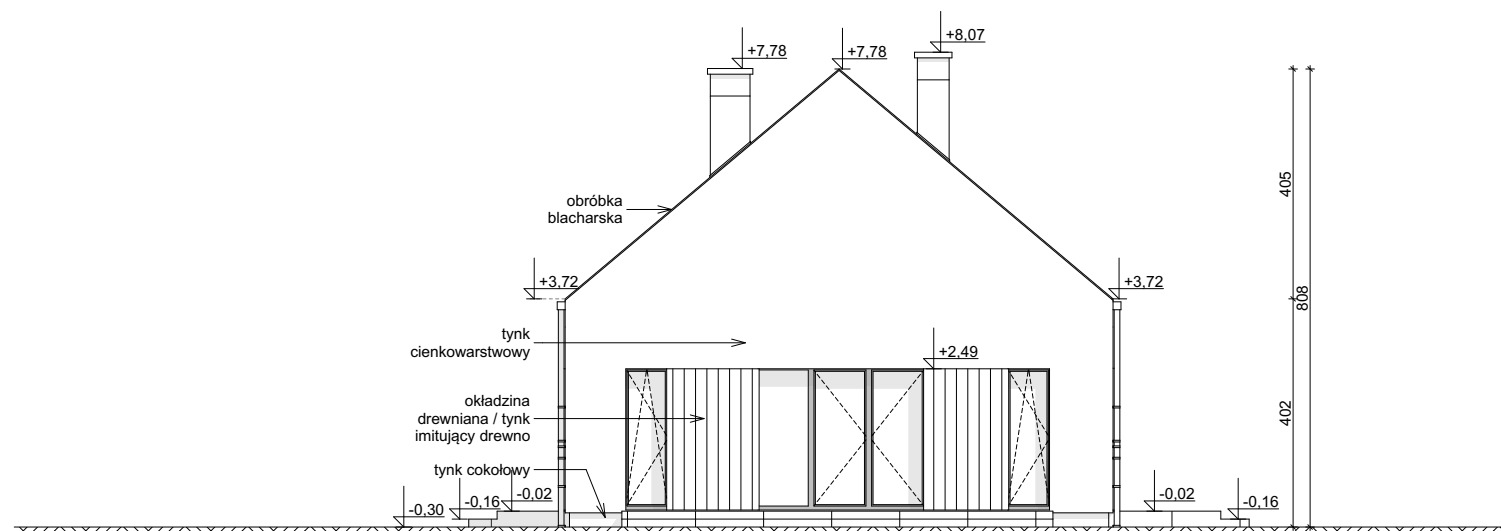
ELEWACJA OGRODOWA
