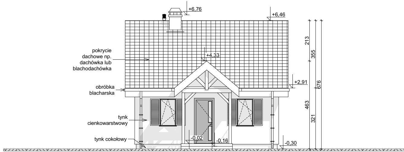
ELEWACJA FRONTOWA
