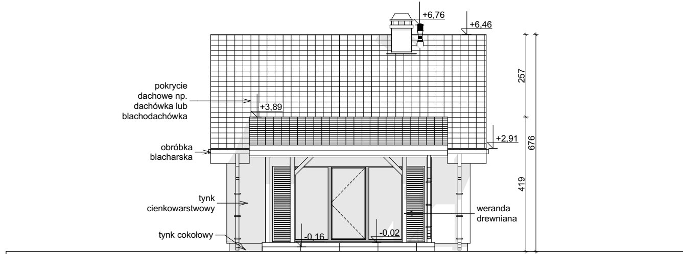
ELEVACJA OGRODOWA
