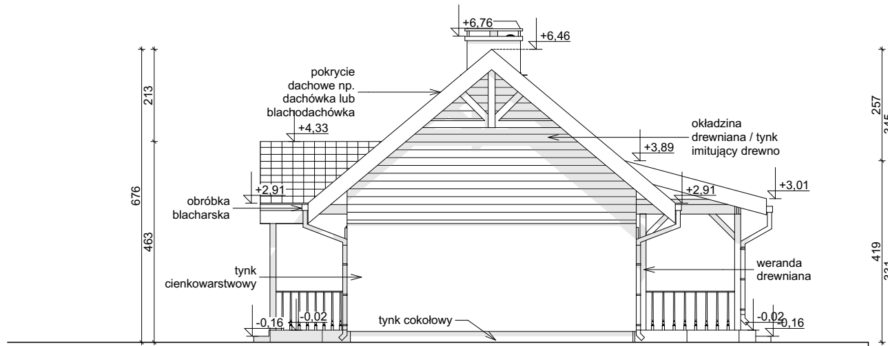
ELEVACJA BOCZNA
