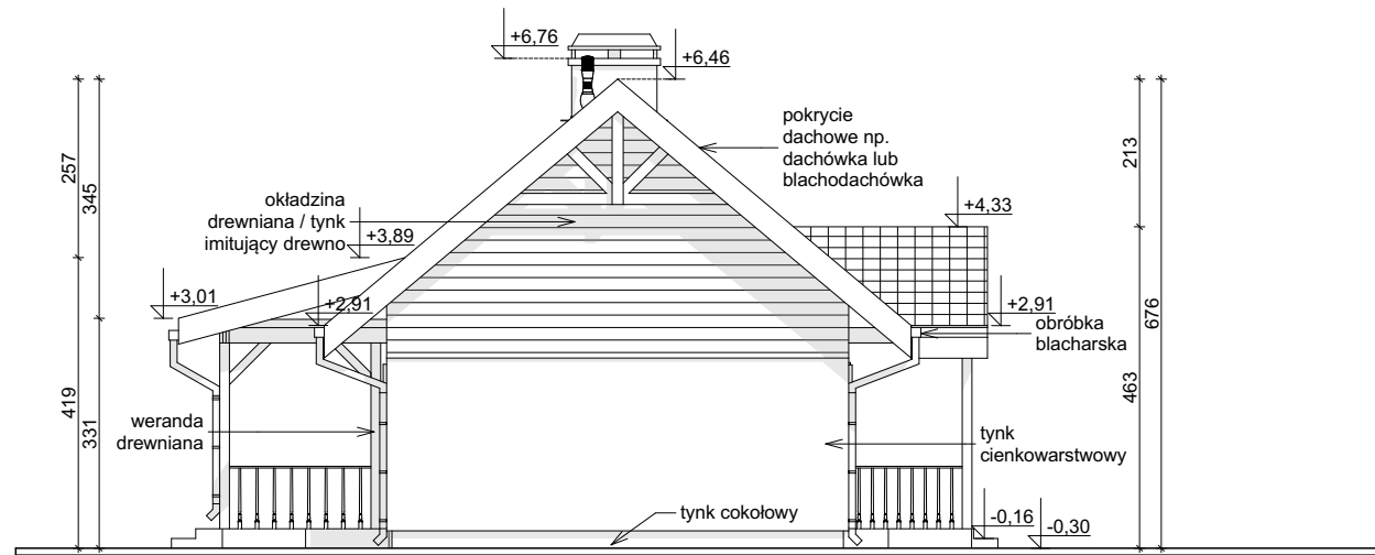
ELEWACJA BOCZNA
