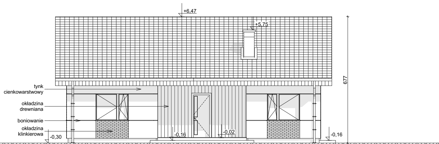
ELEWACJA FRONTOWA
