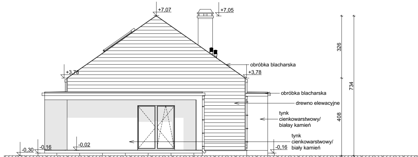
ELEWACJA BOCZNA
