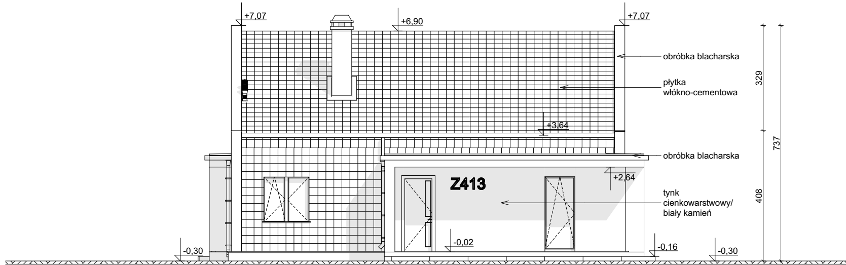
ELEWACJA FRONTOWA
