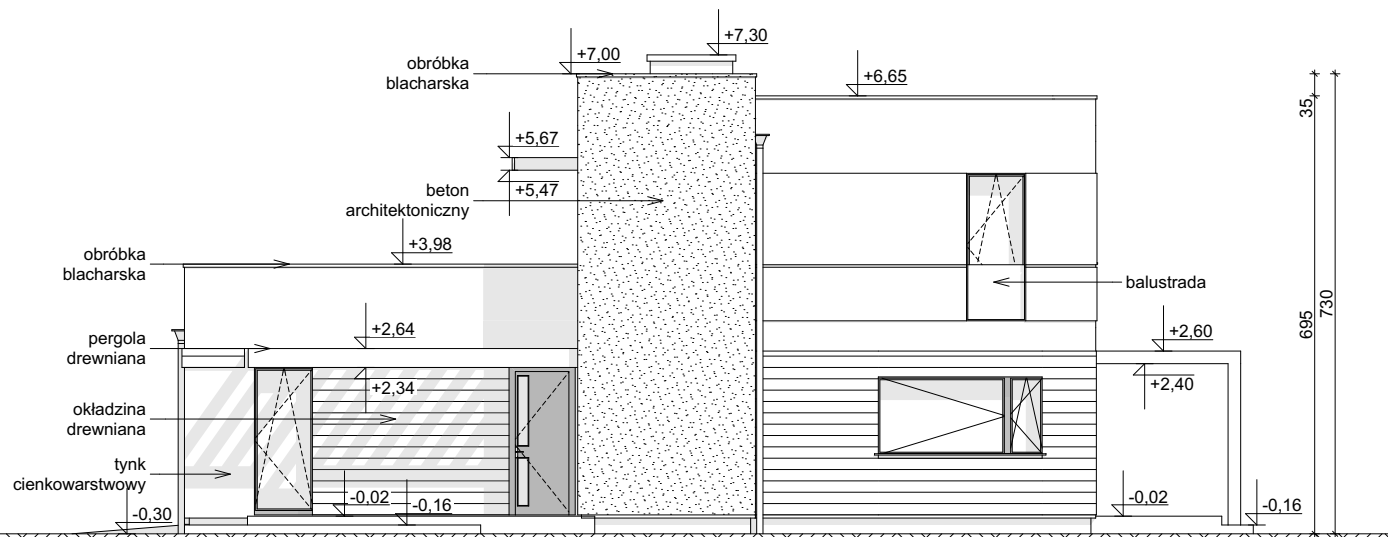
ELEWACJA FRONTOWA
