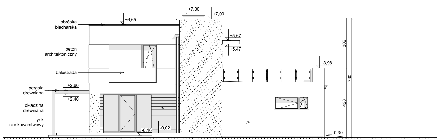
ELEWACJA OGRODOWA
