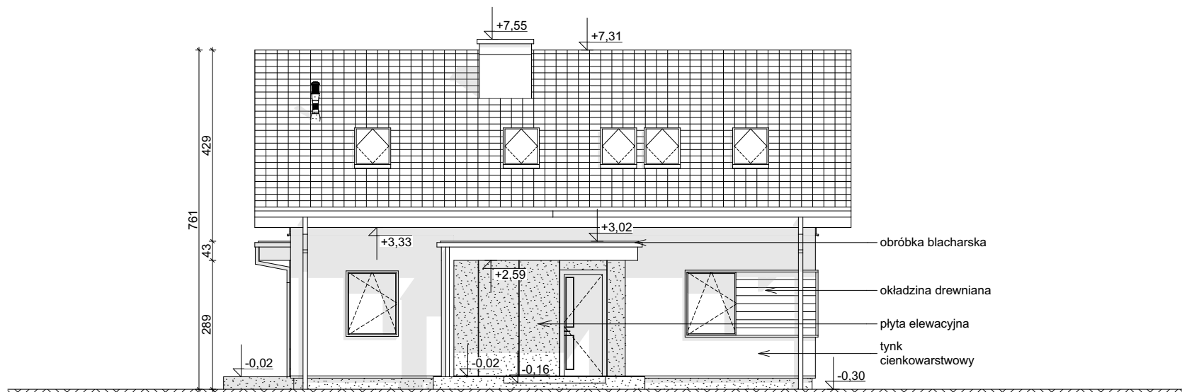
ELEWACJA FRONTOWA
