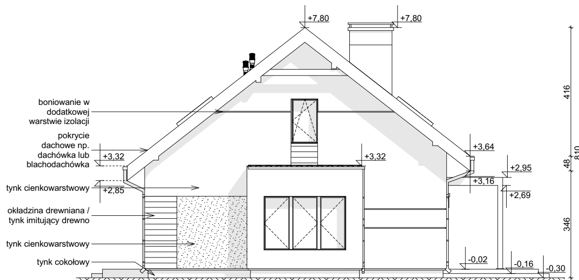
ELEWACJA BOCZNA
