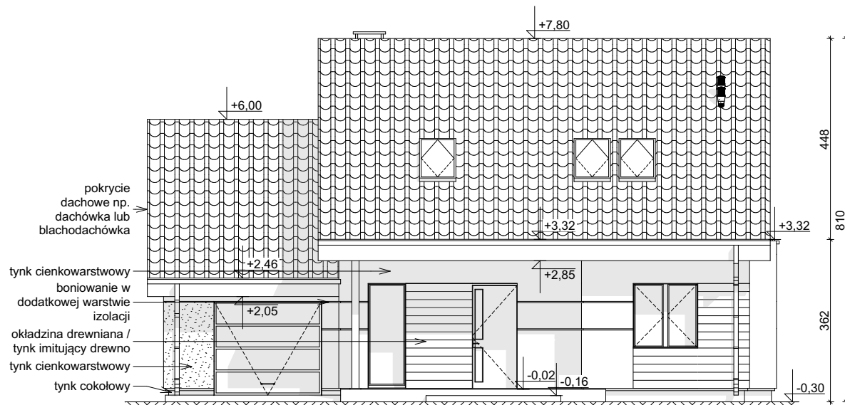
ELEWACJA FRONTOWA
