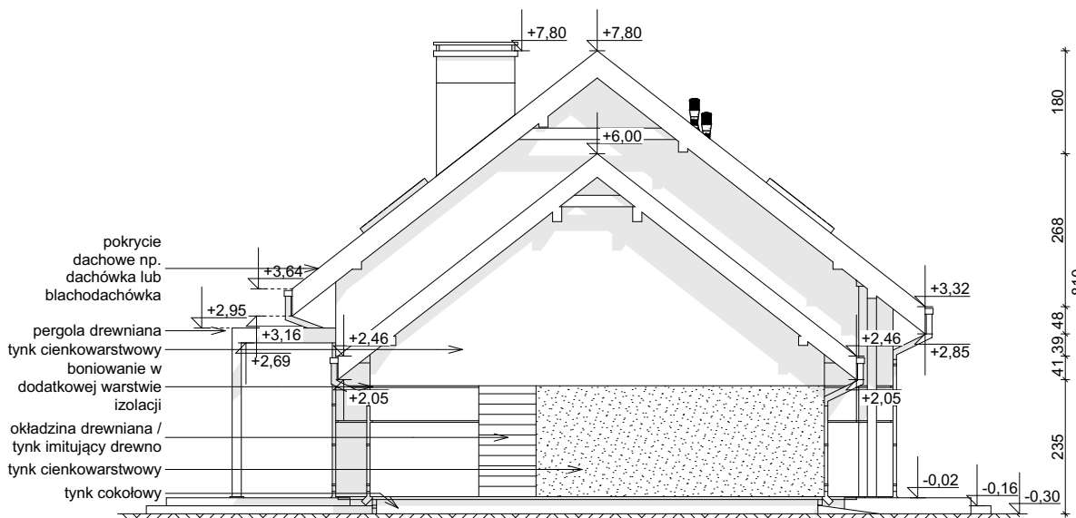
ELEWACJA BOCZNA
