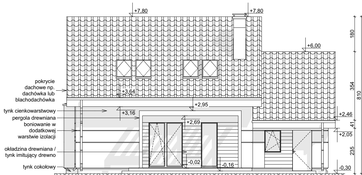
ELEWACJA OGRODOWA
