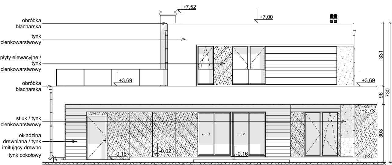
ELEWACJA OGRODOWA
