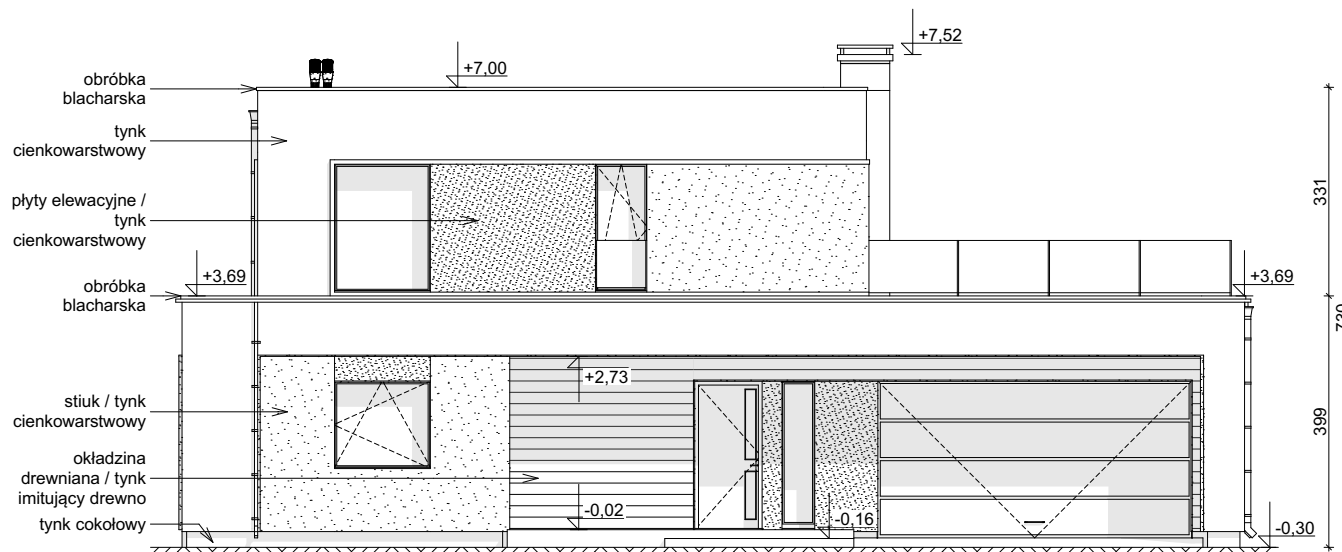
ELEWACJA FRONTOWA
