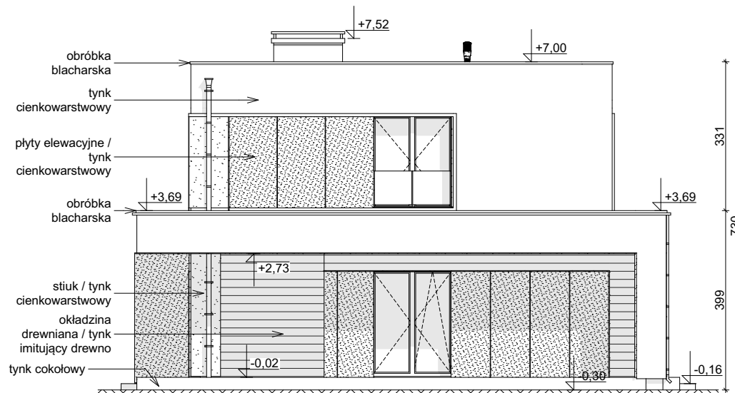
ELEWACJA BOCZNA
