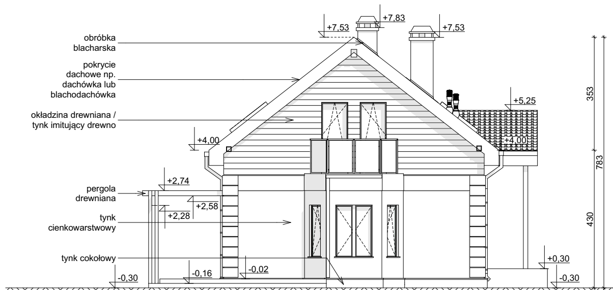
ELEWACJA BOCZNA
