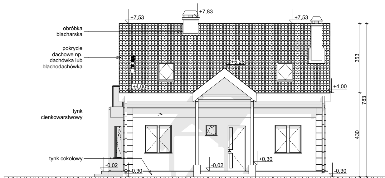
ELEWACJA FRONTOWA
