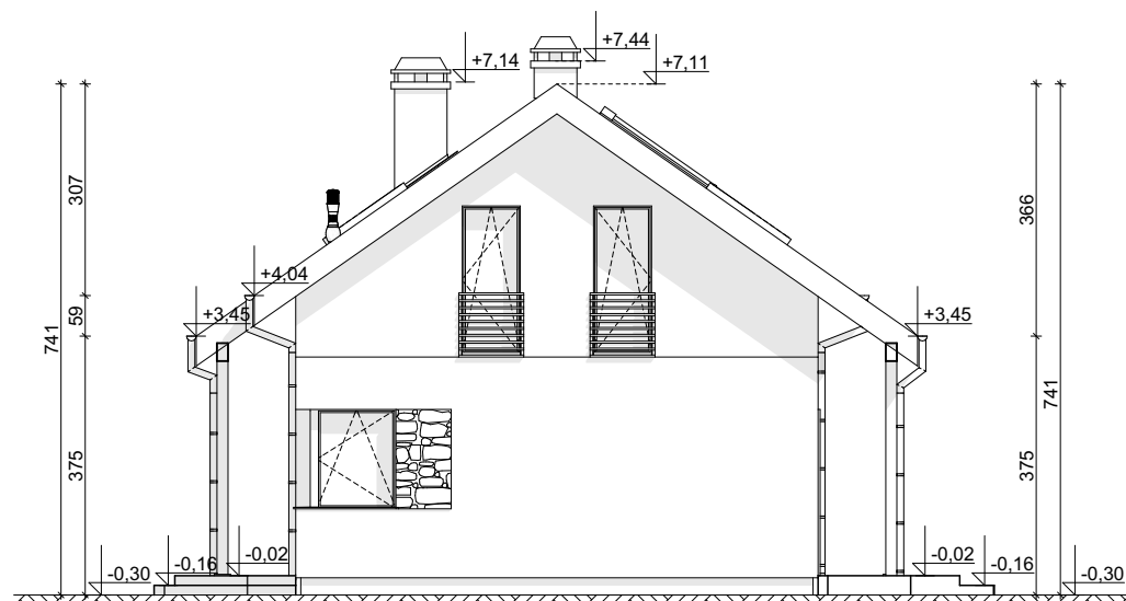
ELEWACJA BOCZNA
