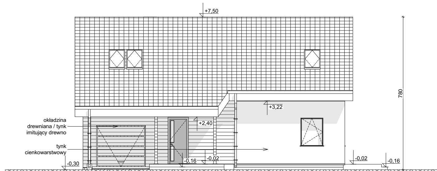
ELEWACJA FRONTOWA
