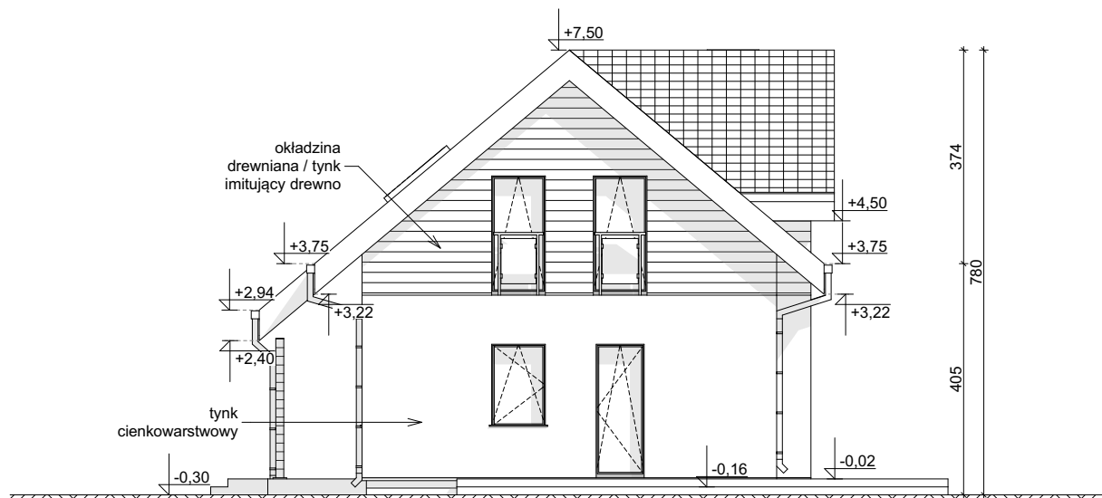
ELEWACJA BOCZNA
