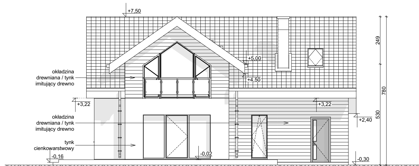
ELEWACJA OGRODOWA
