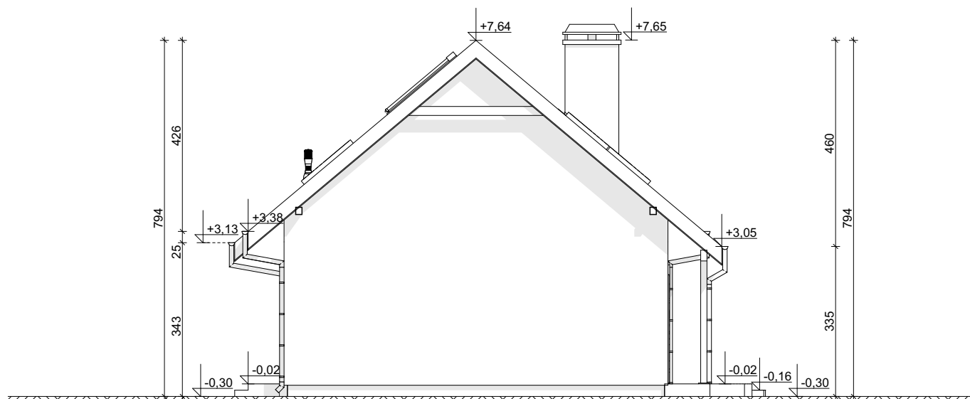
ELEVACJA BOCZNA
