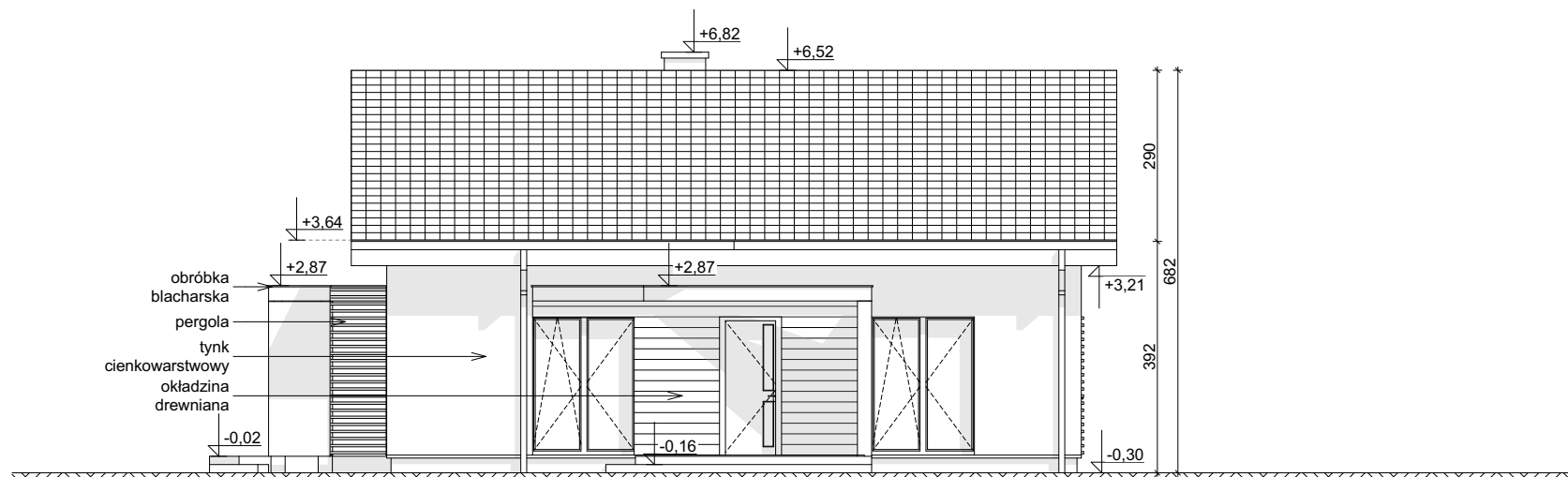
ELEWACJA FRONTOWA
