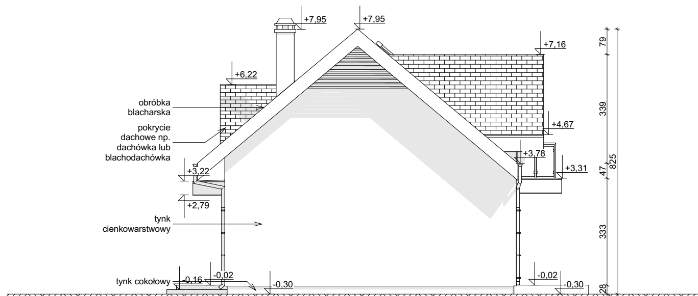
ELEVACJA BOCZNA
