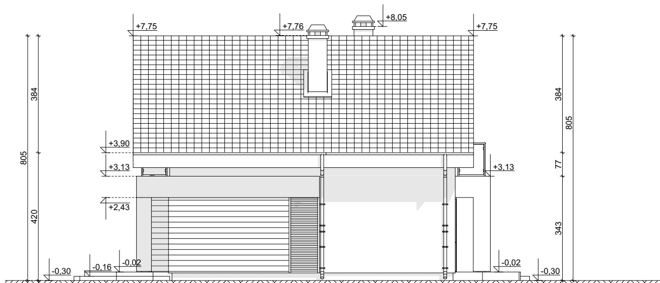
ELEVACJA BOCZNA
