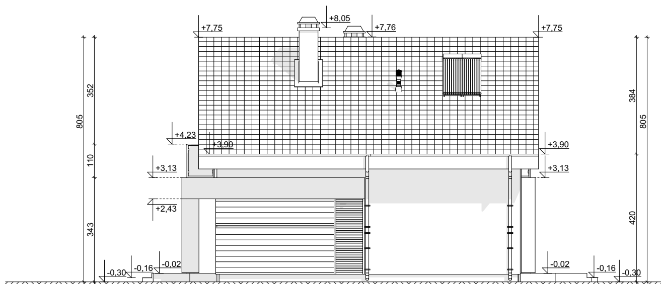
ELEVACJA BOCZNA
