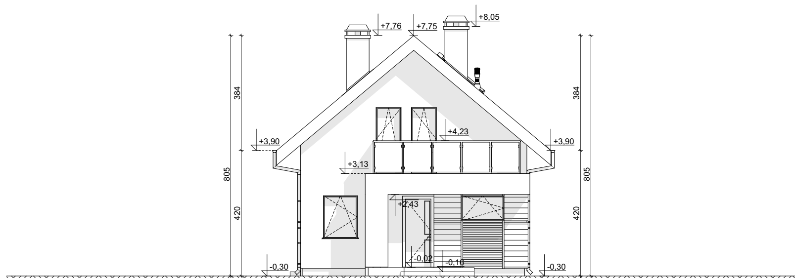
ELEVACJA FRONTOWA
