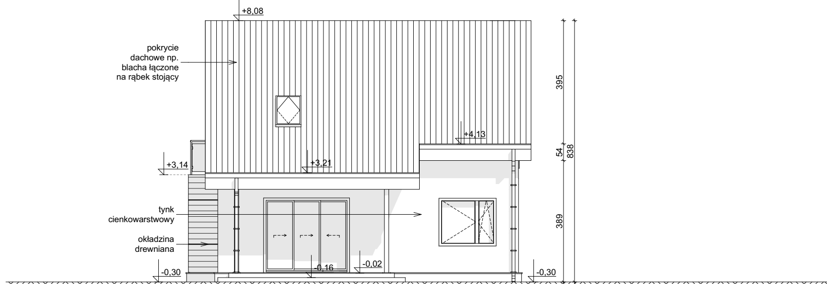
ELEWACJA OGRODOWA
