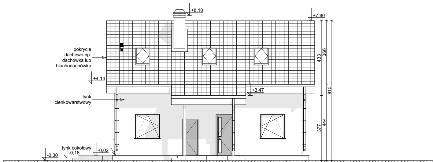
ELEWACJA FRONTOWA
