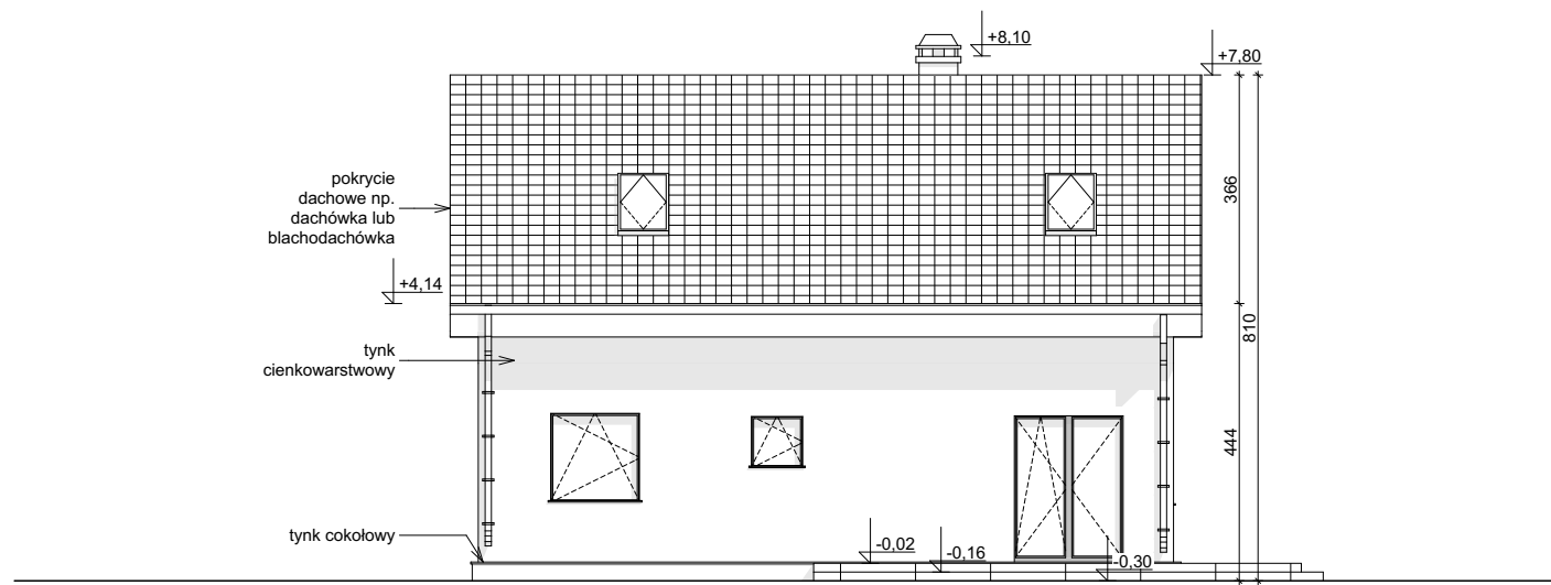
ELEWACJA OGRODOWA
