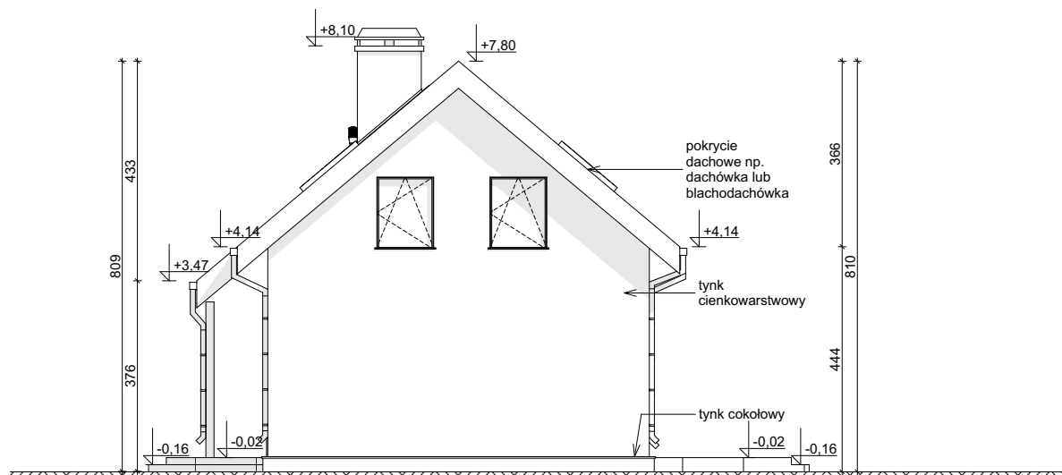
ELEWACJA BOCZNA
