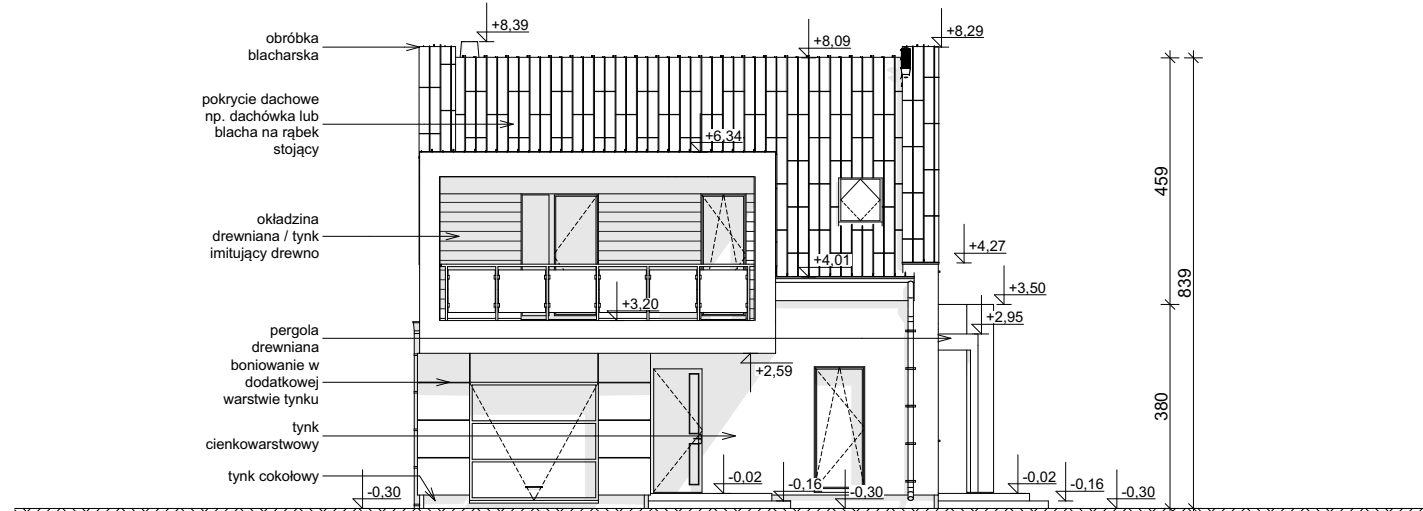
ELEWACJA FRONTOWA
