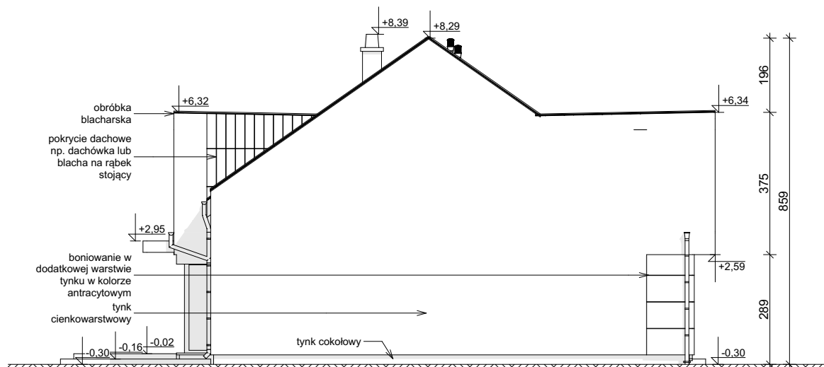
ELEWACJA BOCZNA
