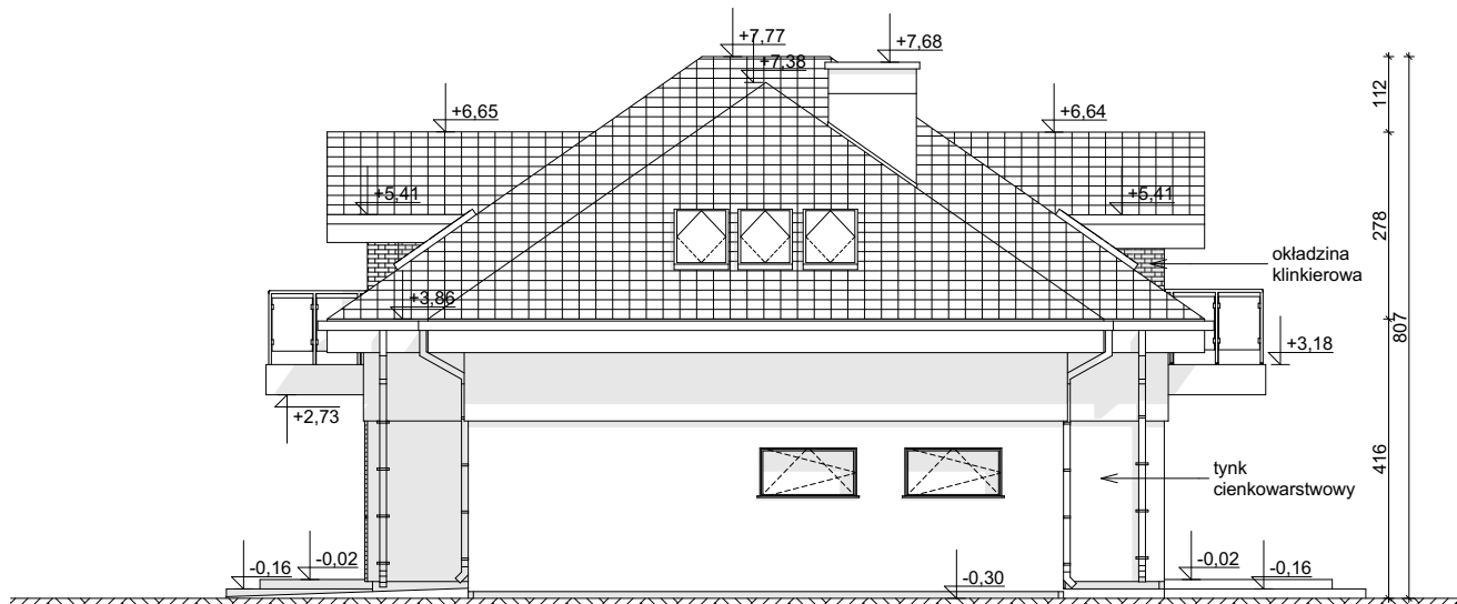
ELEWACJA BOCZNA
