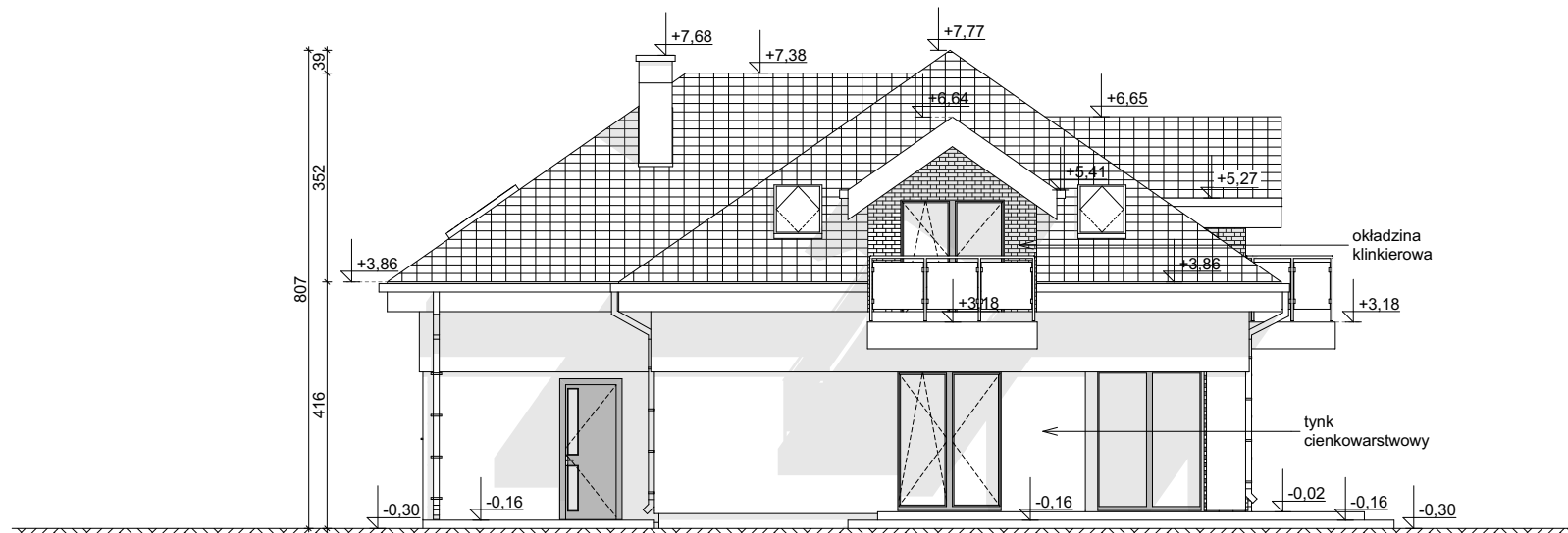
ELEWACJA OGRODOWA
