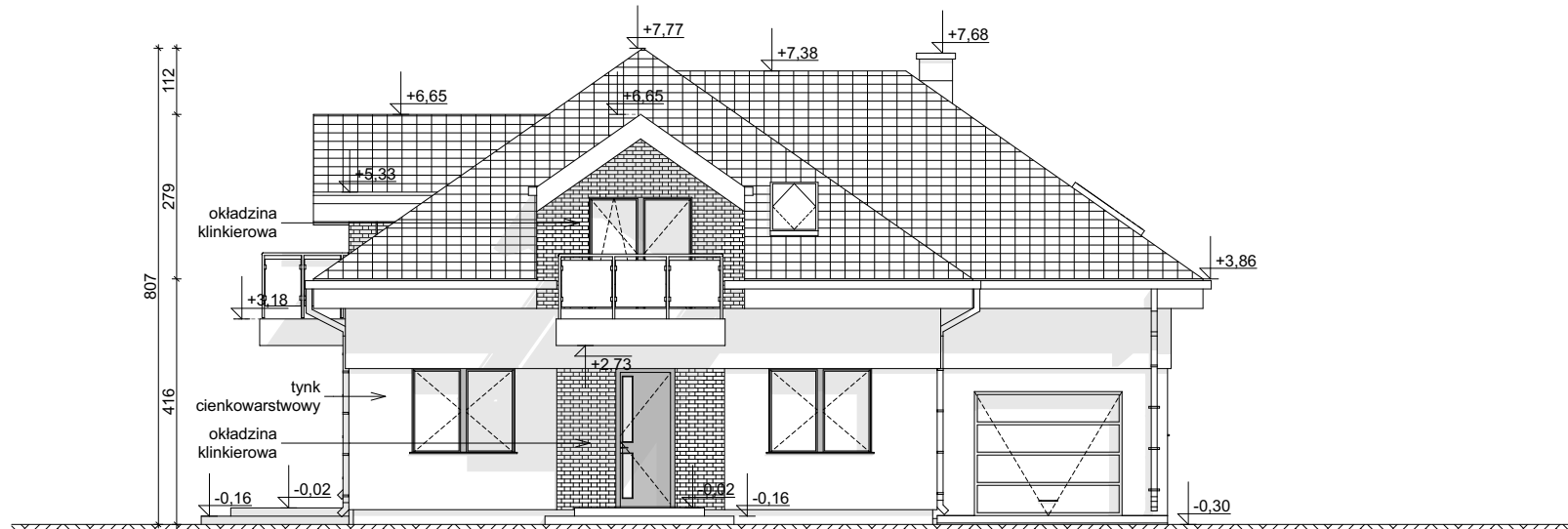
ELEWACJA FRONTOWA
