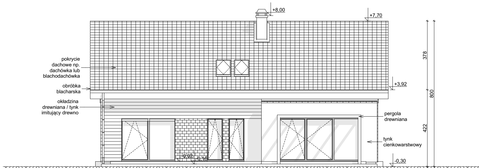
ELEWACJA OGRODOWA
