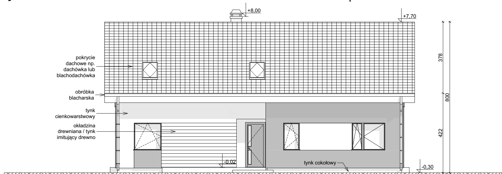
ELEWACJA FRONTOWA
