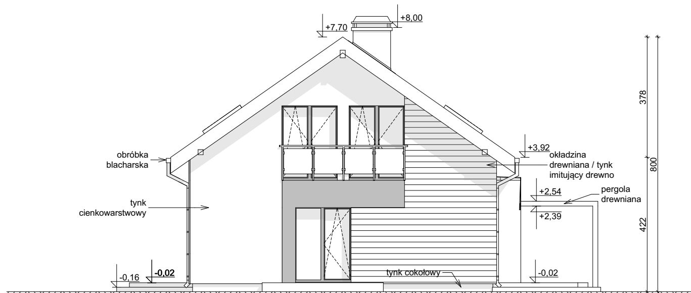
ELEWACJA BOCZNA
