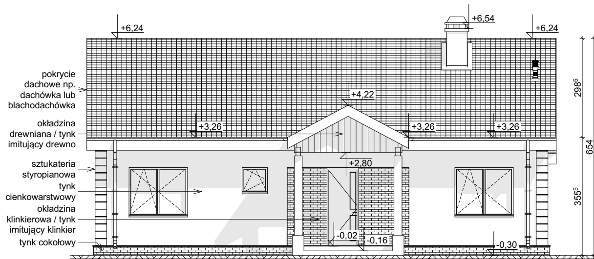
ELEWACJA FRONTOWA
