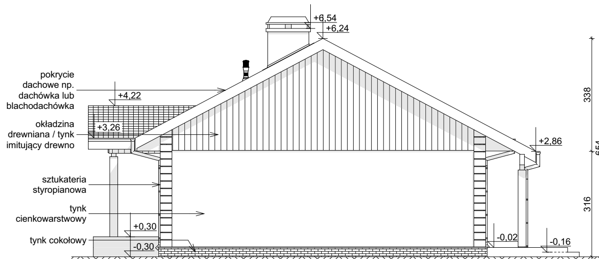
ELEWACJA BOCZNA
