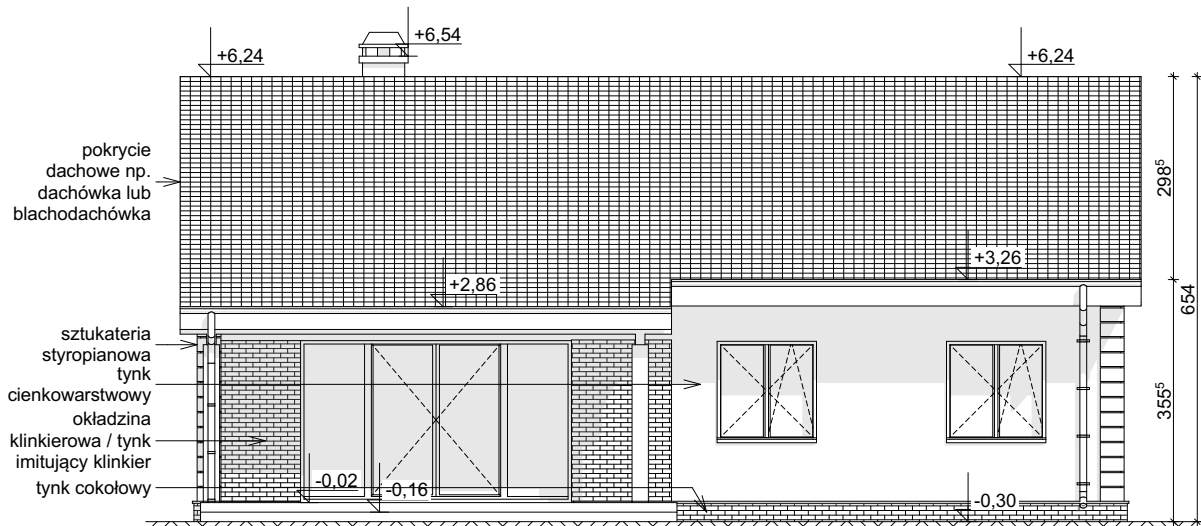
ELEWACJA OGRODOWA
