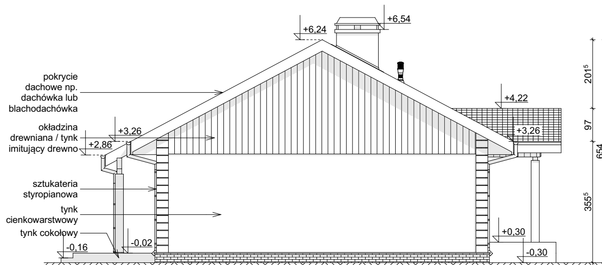
ELEWACJA BOCZNA
