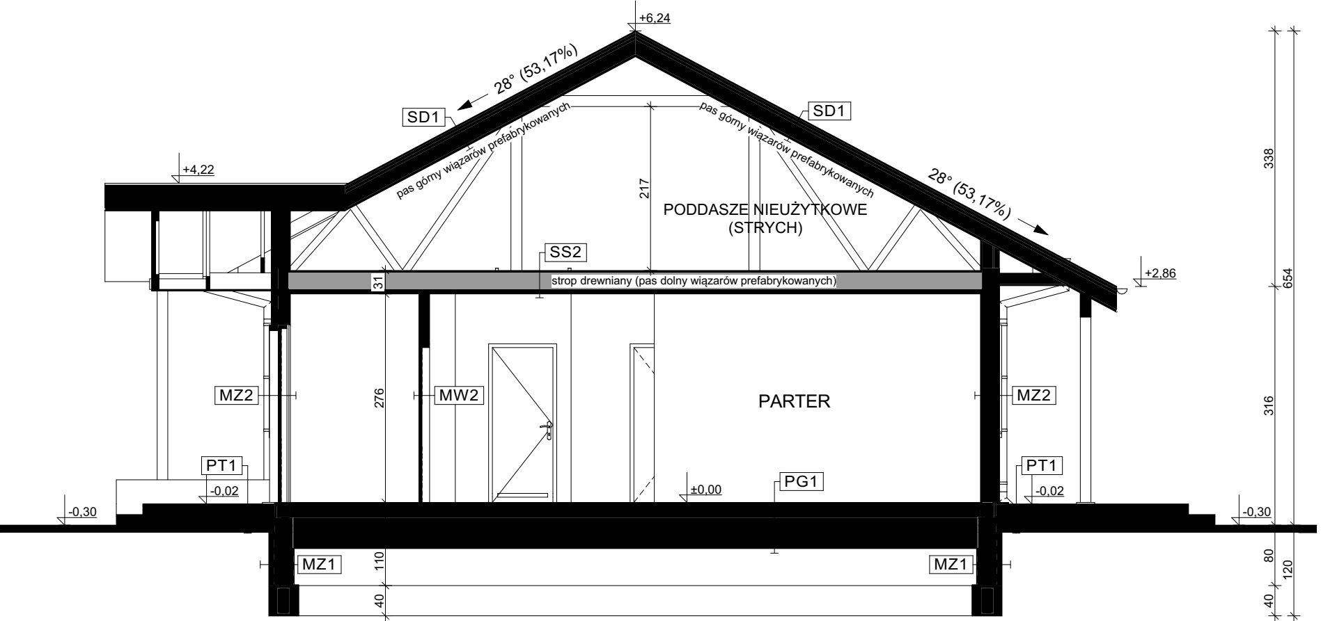
PRZEKRÓJ B-B
