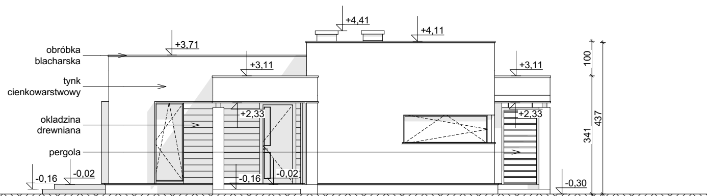
ELEWACJA FRONTOWA
