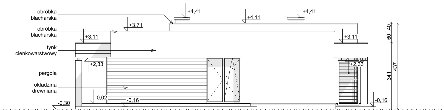
ELEWACJA BOCZNA
