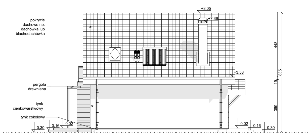
ELEWACJA BOCZNA
