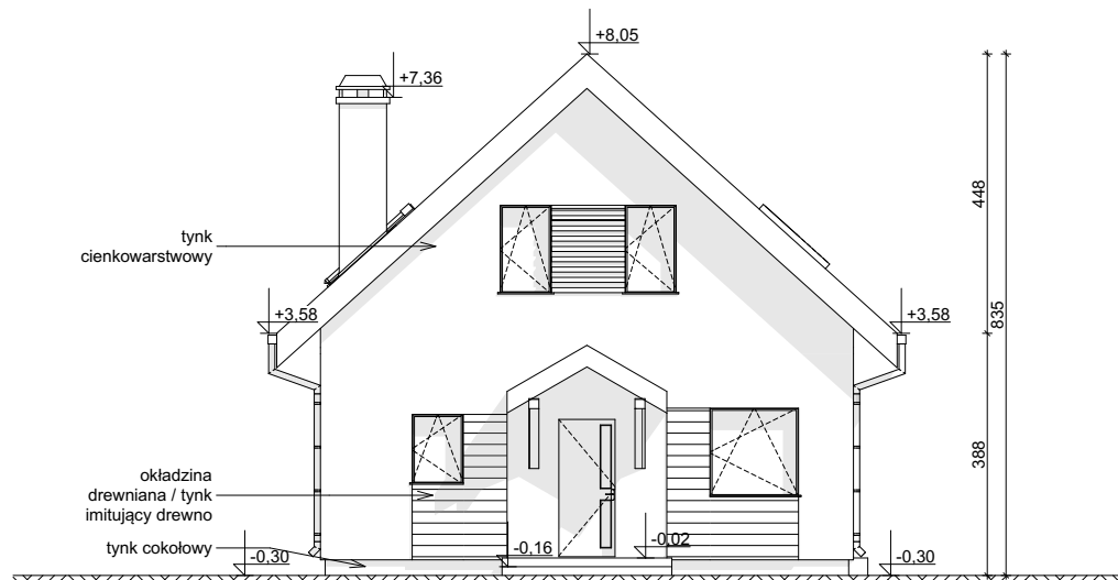
ELEWACJA FRONTOWA
