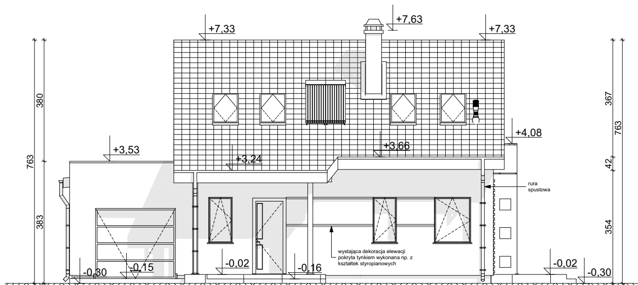
ELEWACJA FRONTOWA
