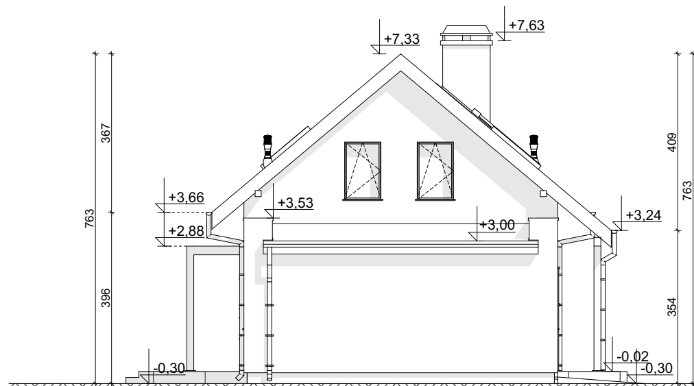
ELEWACJA BOCZNA
