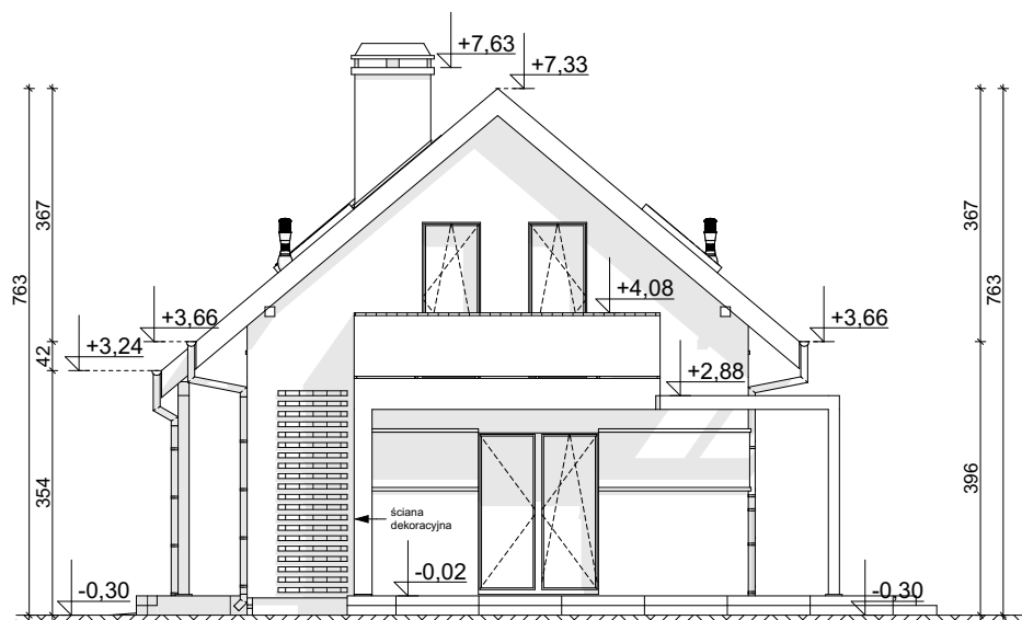
ELEVACJA BOCZNA
