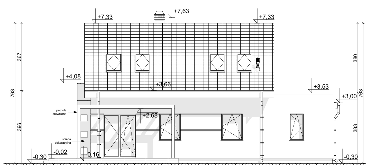
ELEVACJA OGRODOWA
