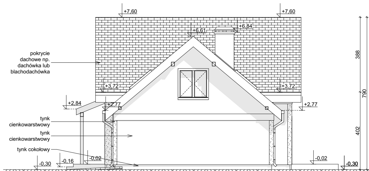
ELEWACJA BOCZNA
