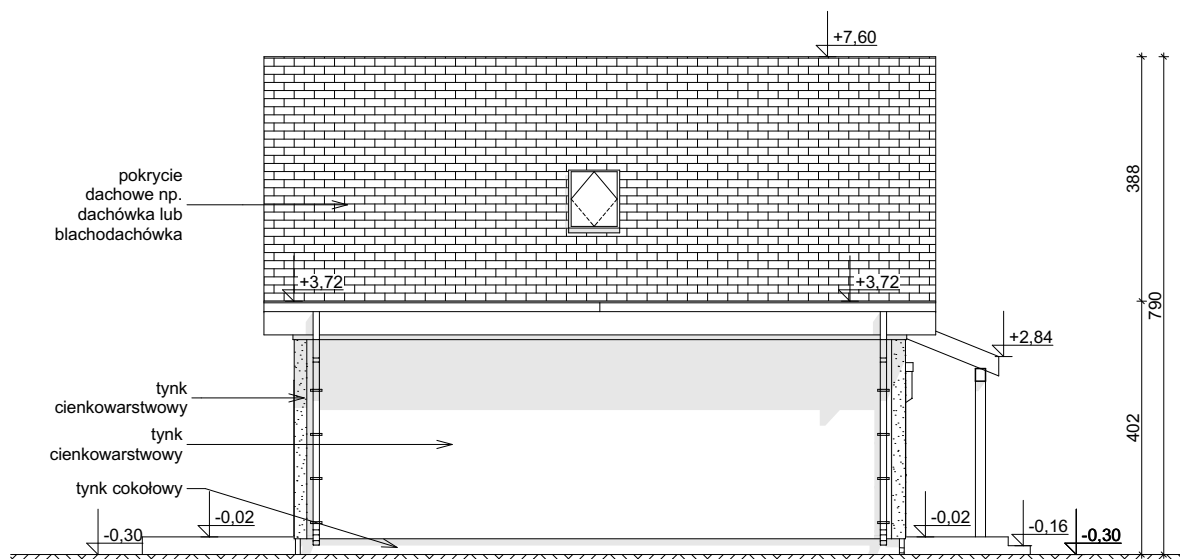
ELEWACJA BOCZNA
