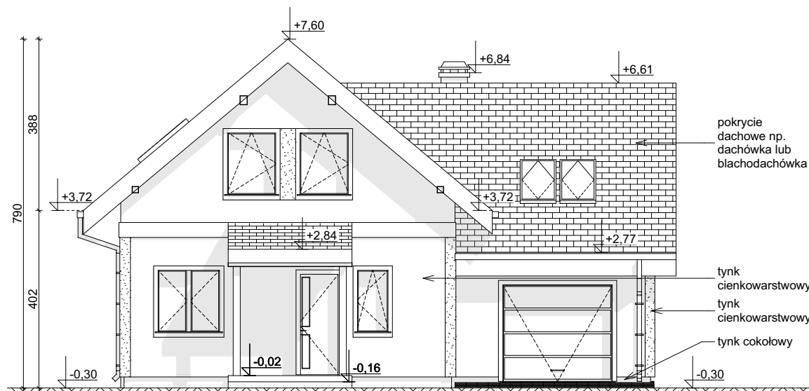
ELEWACJA FRONTOWA
