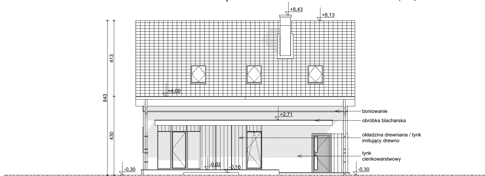
ELEWACJA OGRODOWA
