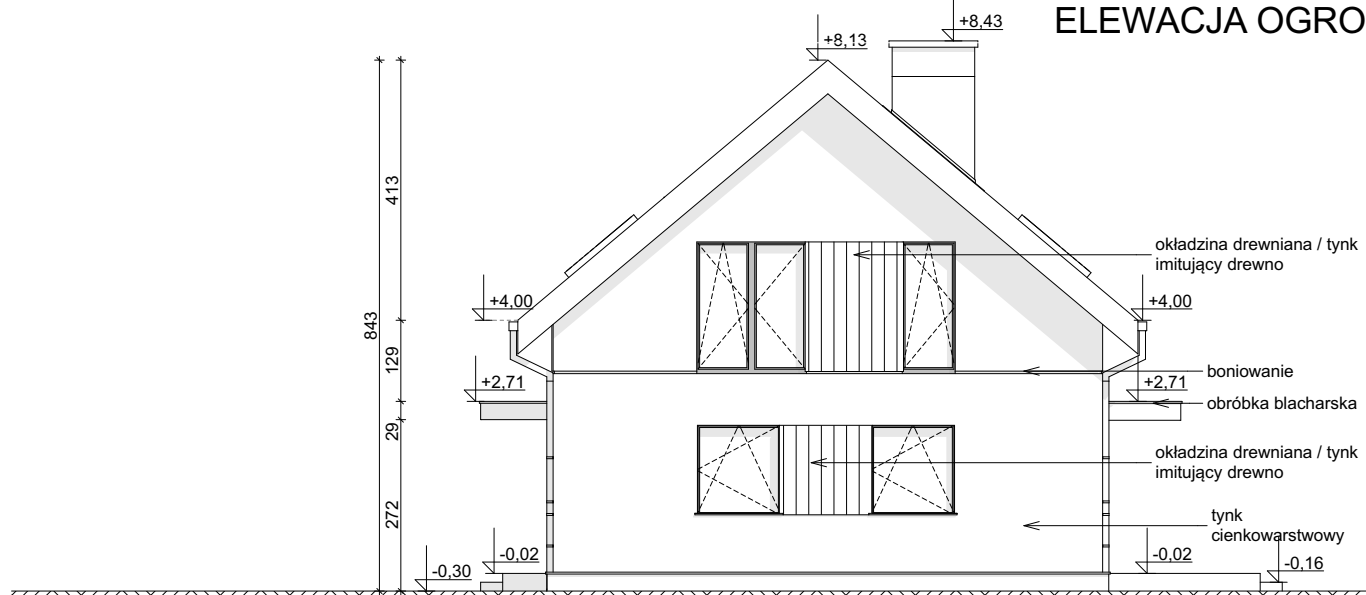
ELEWACJA BOCZNA
