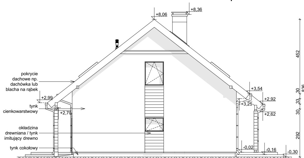
ELEWACJA BOCZNA
