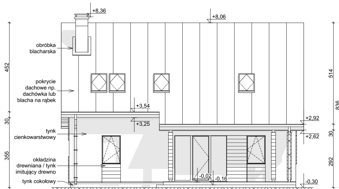
ELEWACJA OGRODOWA
