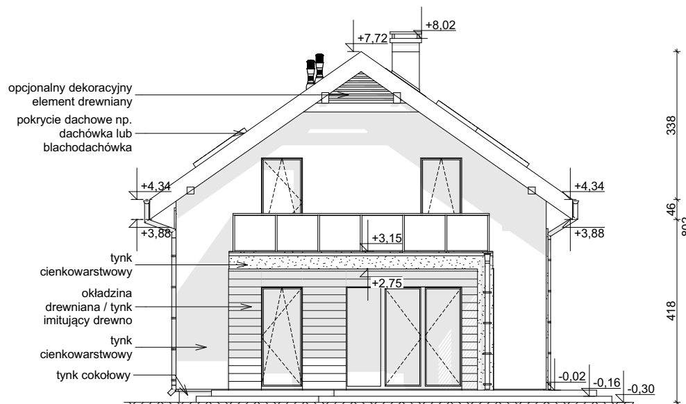
ELEWACJA BOCZNA
