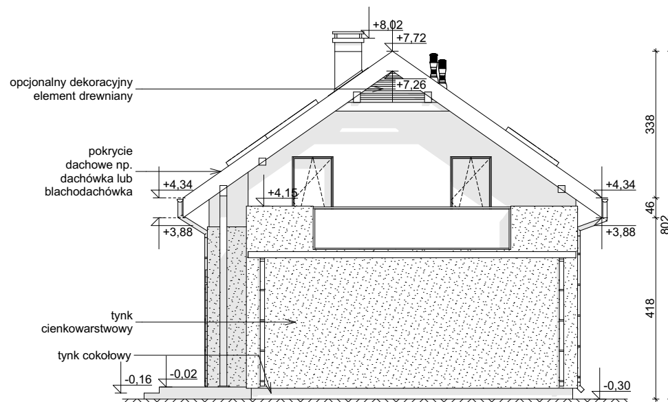
ELEWACJA BOCZNA
