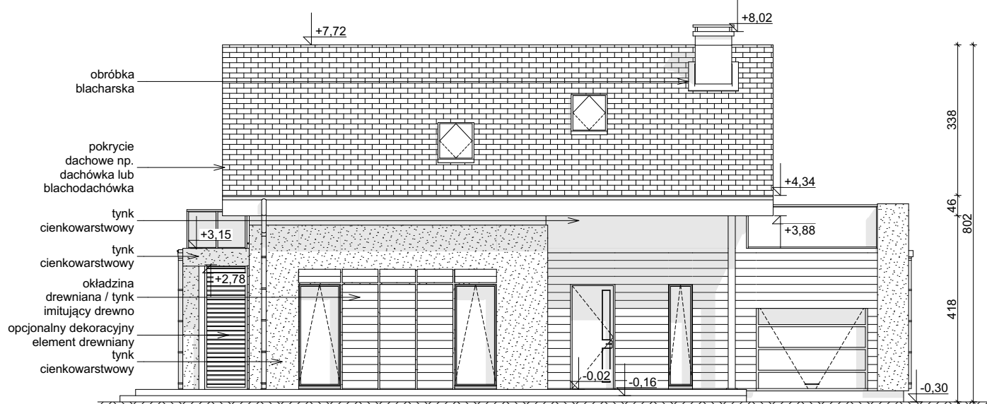
ELEWACJA FRONTOWA
