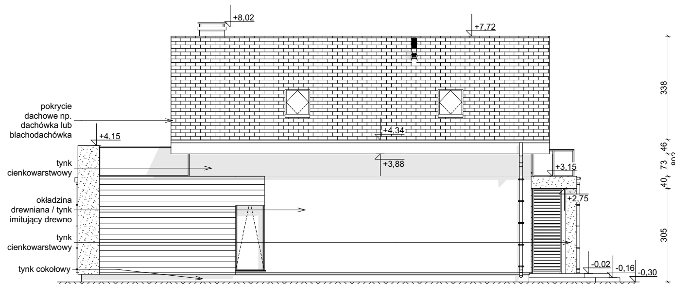
ELEWACJA OGRODOWA
