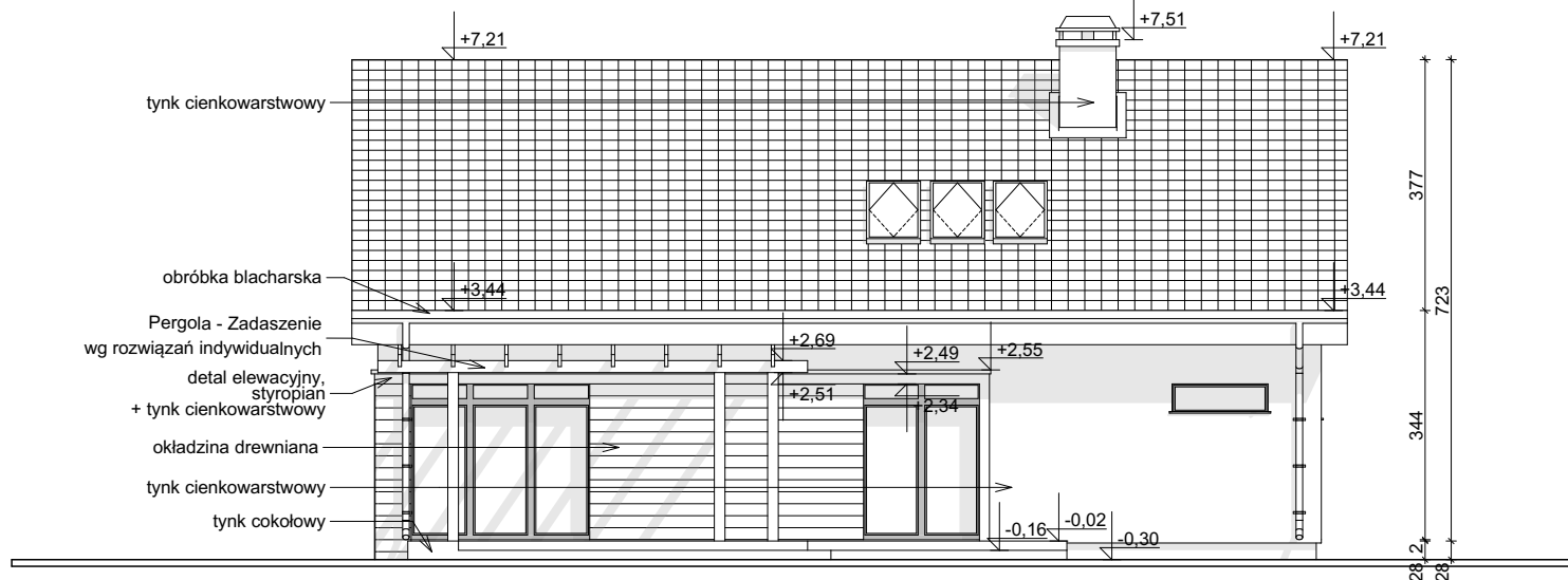
ELEWACJA OGRODOWA
