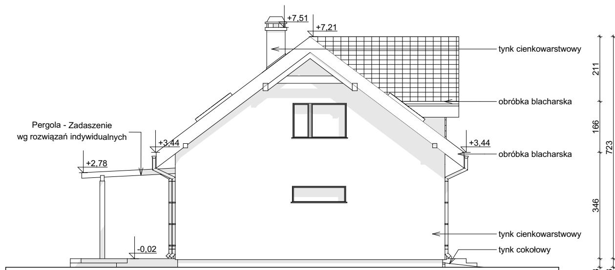
ELEWACJA BOCZNA
