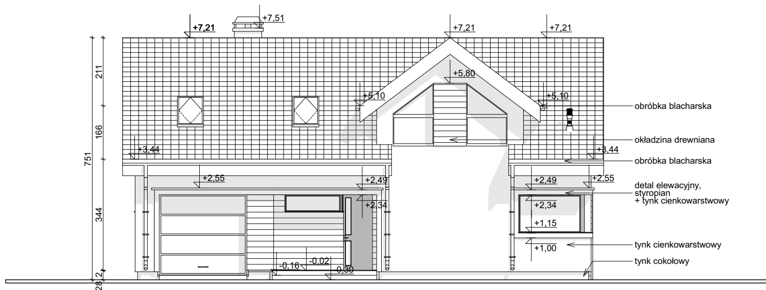
ELEWACJA FRONTOWA
