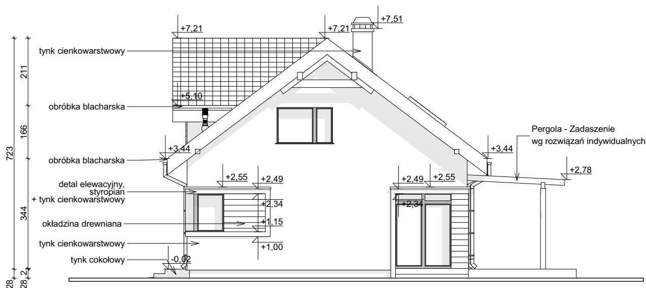
ELEWACJA BOCZNA
