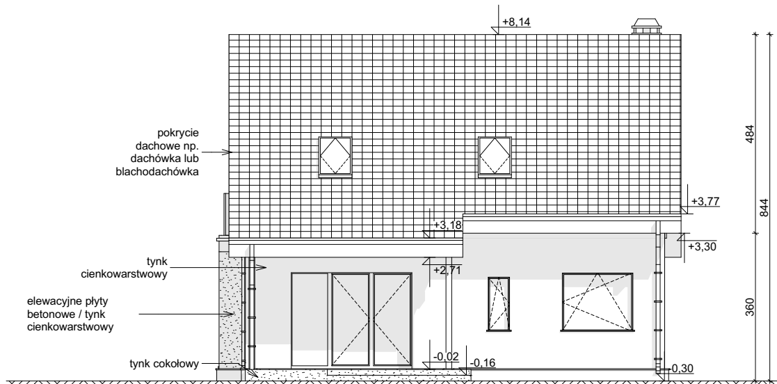
ELEWACJA OGRODOWA
