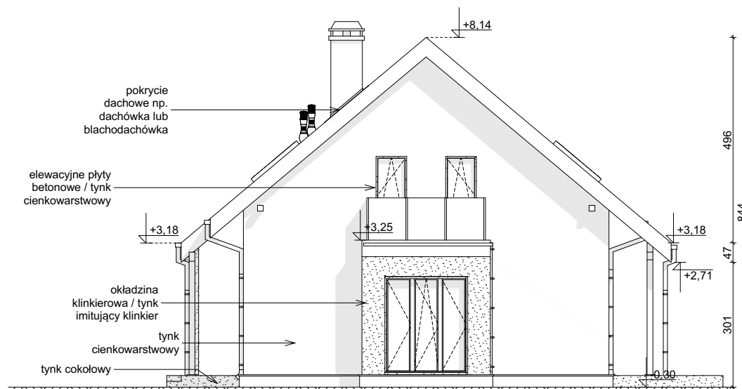
ELEWACJA BOCZNA
