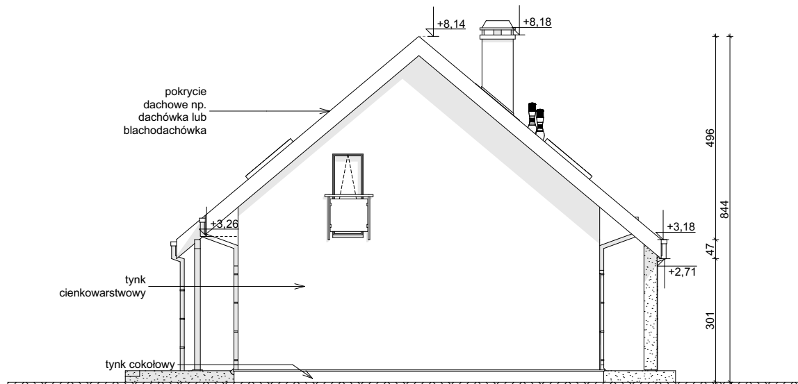
ELEWACJA BOCZNA
