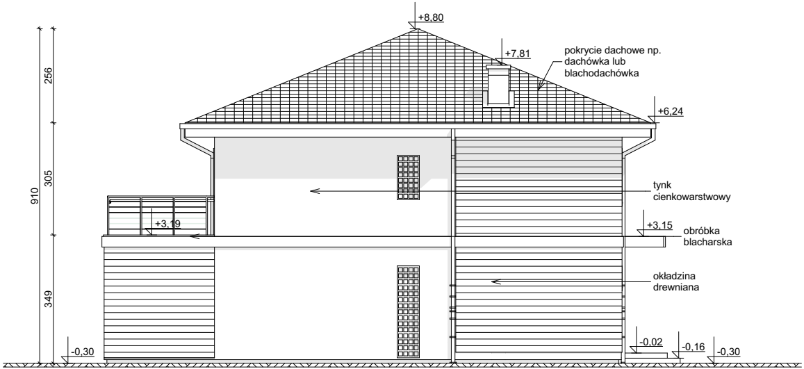
ELEWACJA BOCZNA
