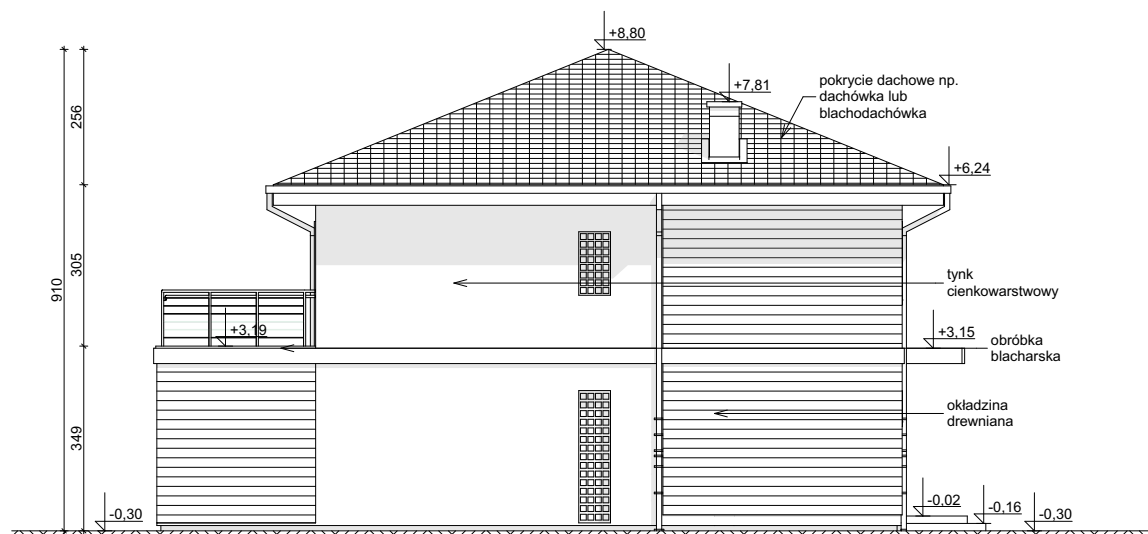
ELEWACJA BOCZNA
