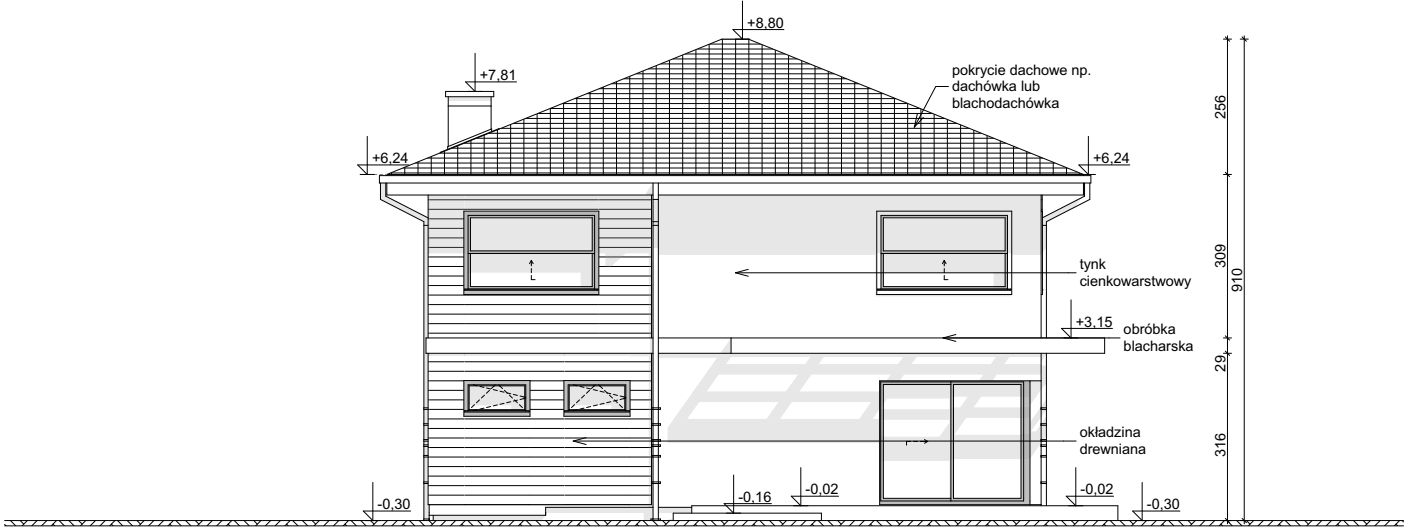
ELEWACJA OGRODOWA
