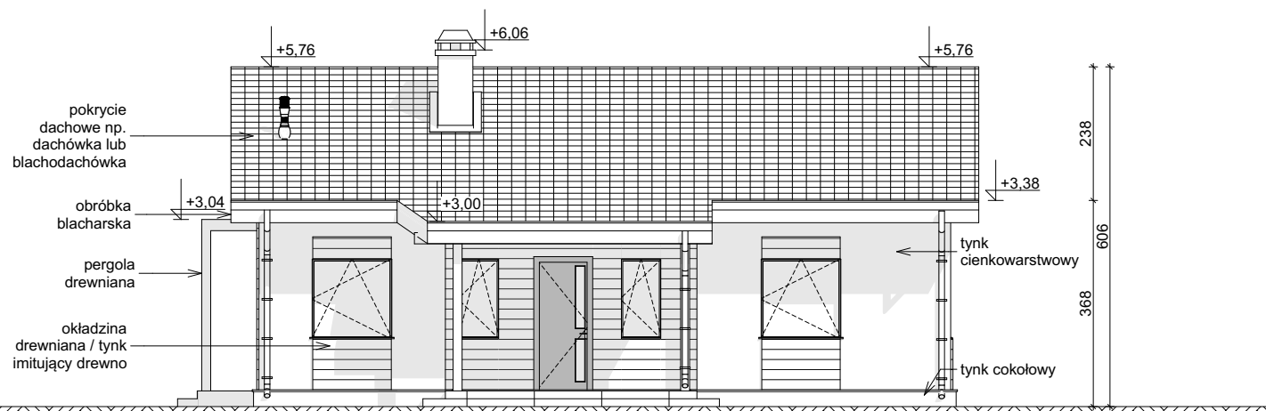
ELEWACJA FRONTOWA
