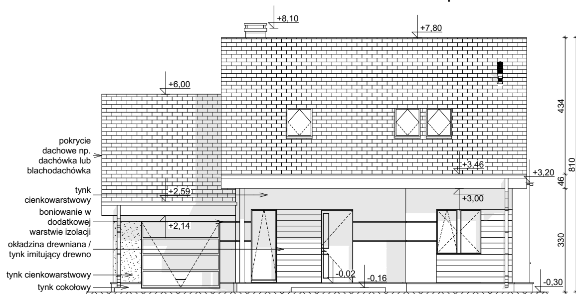
ELEWACJA FRONTOWA
