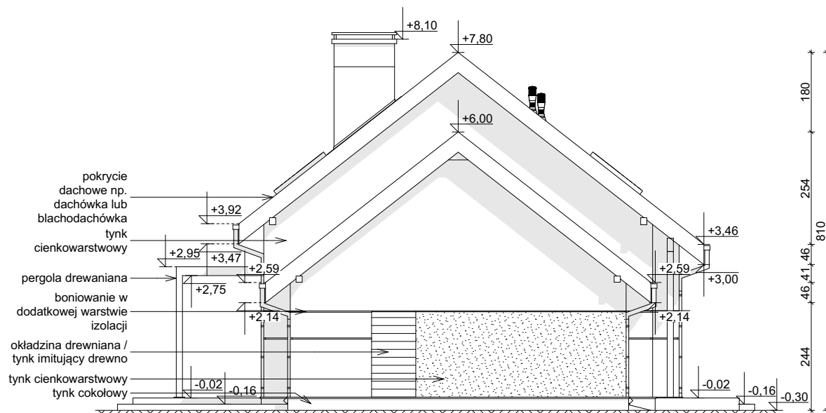
ELEWACJA BOCZNA
