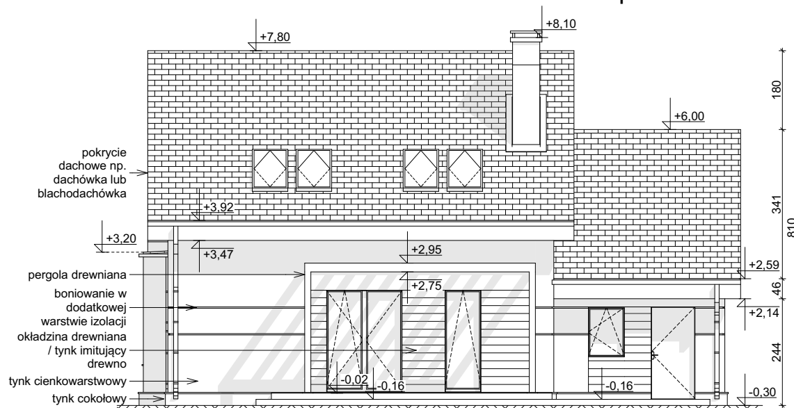
ELEWACJA OGRODOWA
