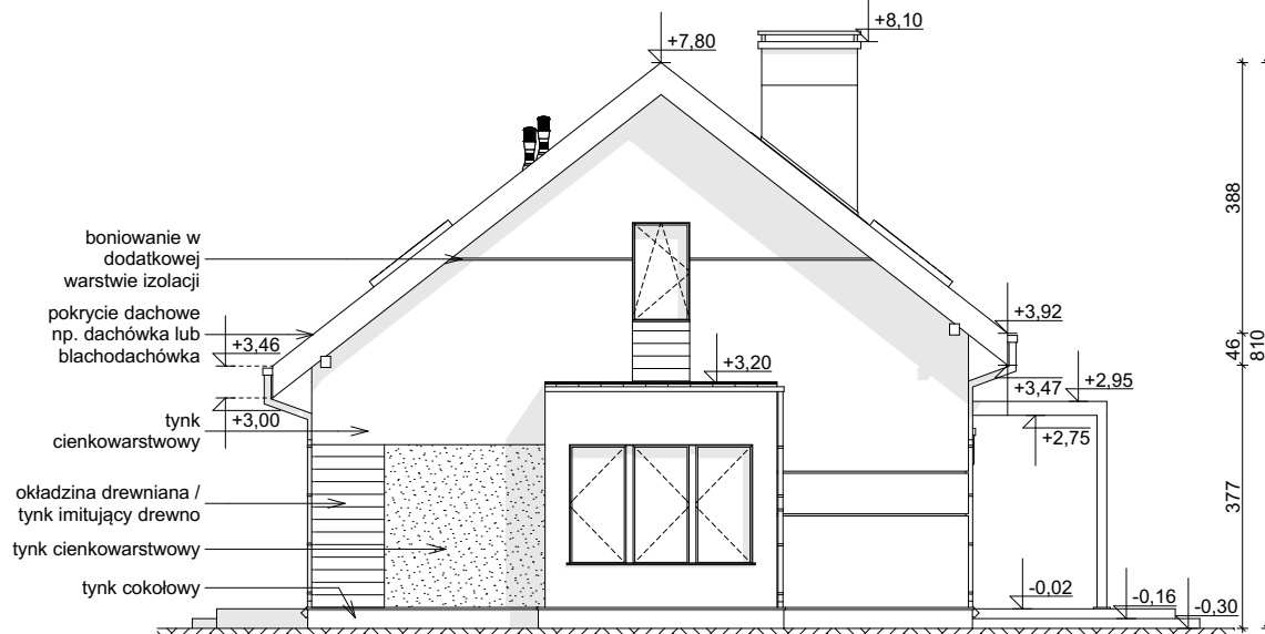
ELEWACJA BOCZNA
