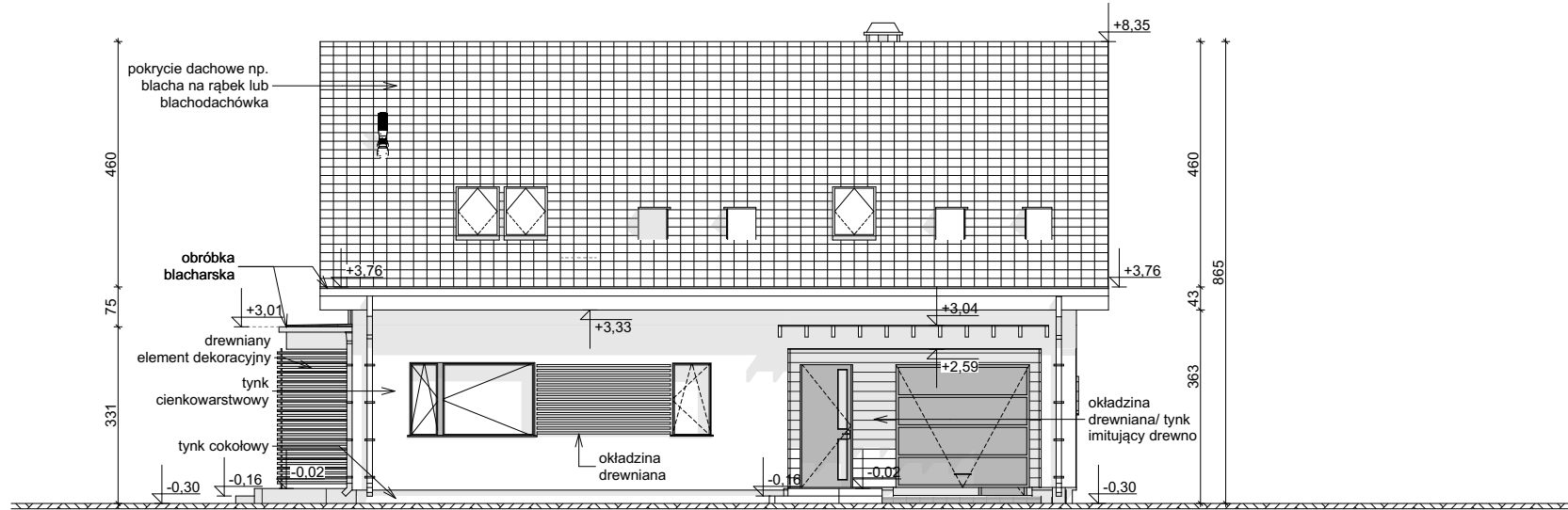
ELEWACJA FRONTOWA
