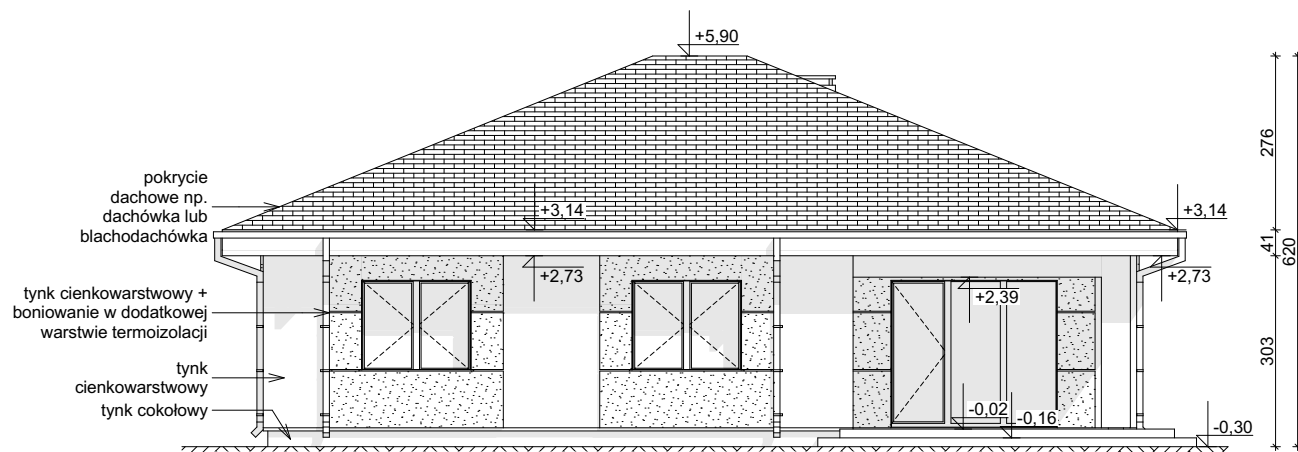
ELEWACJA OGRODOWA
