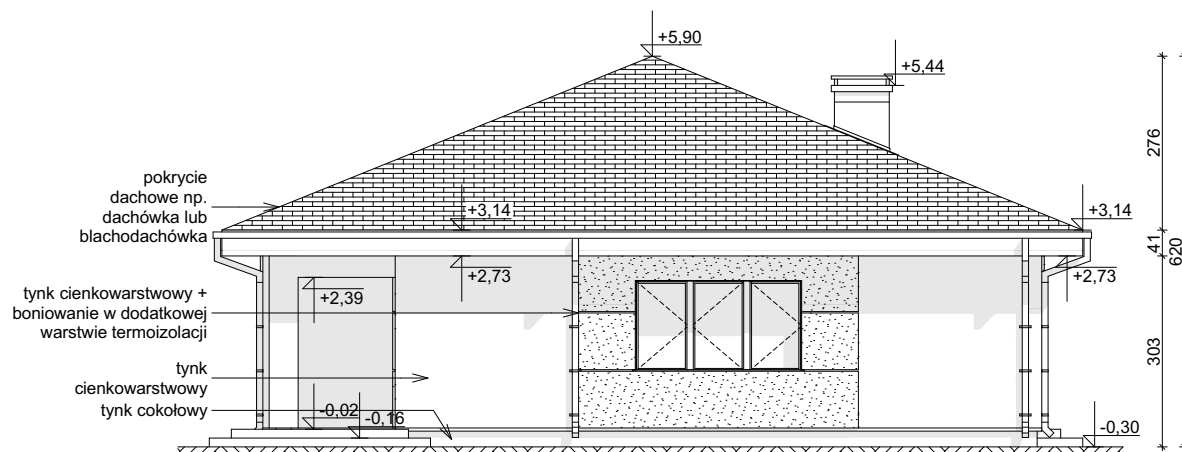
ELEWACJA BOCZNA
