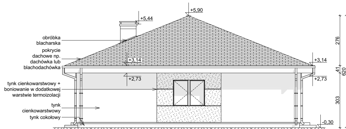
ELEWACJA BOCZNA
