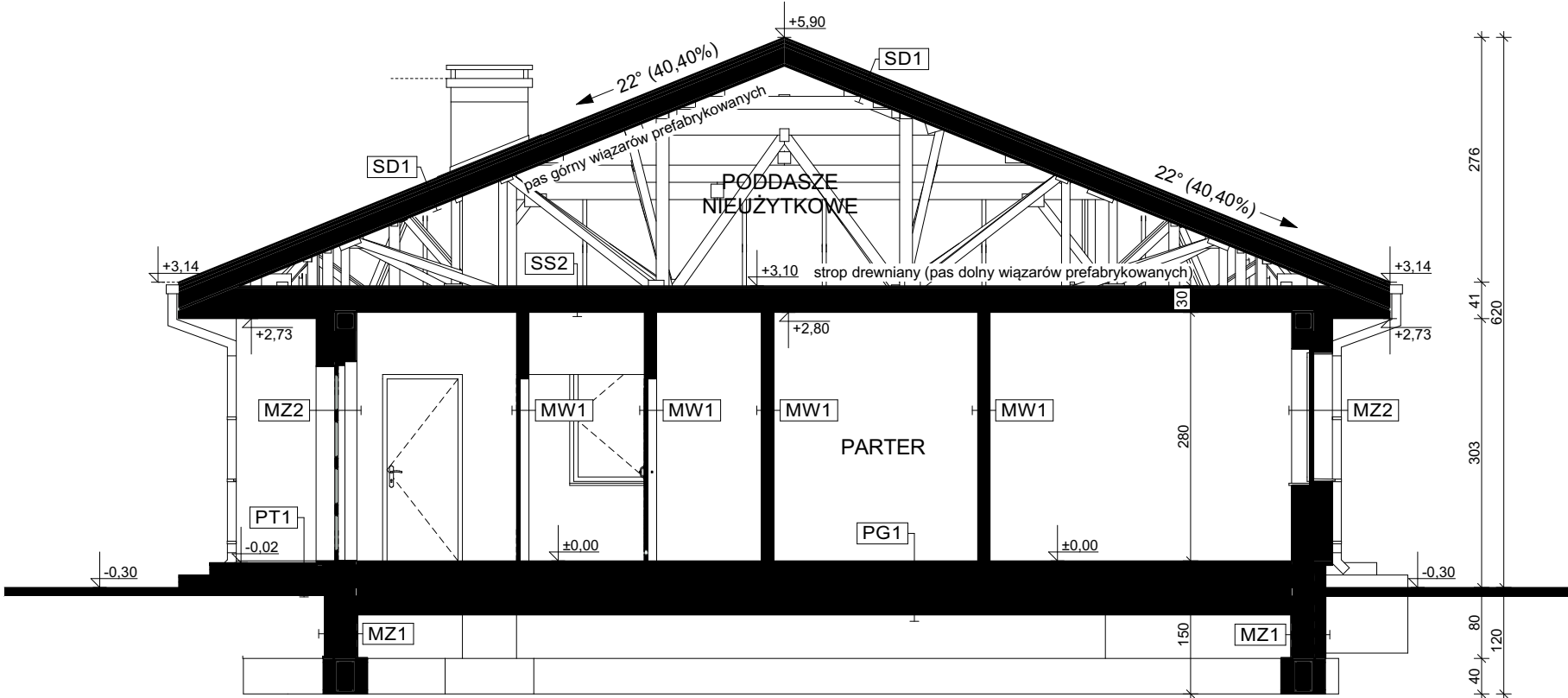
PRZEKRÓJ B-B
