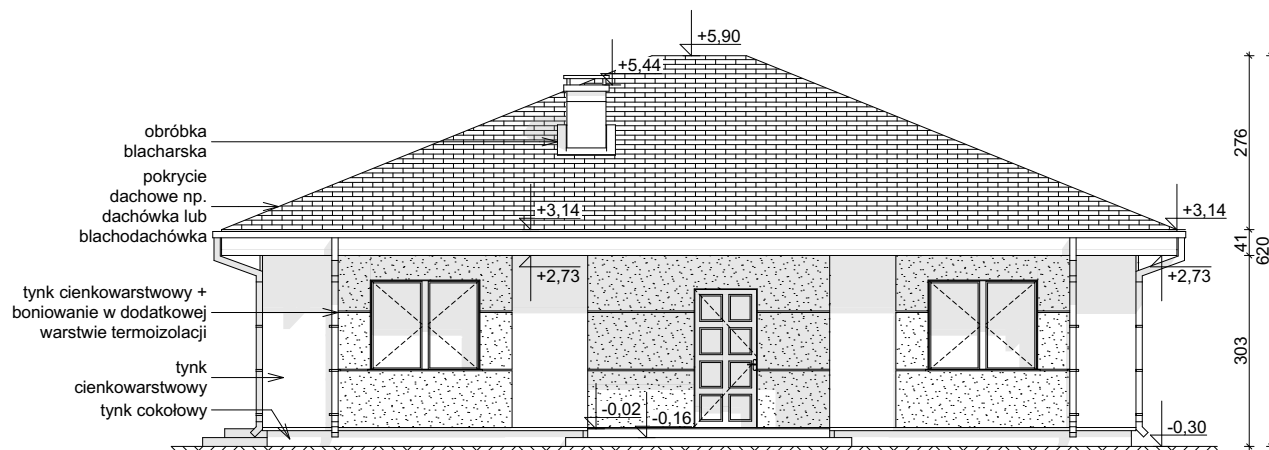
ELEWACJA FRONTOWA
