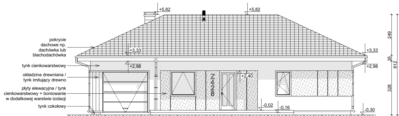
ELEWACJA FRONTOWA
