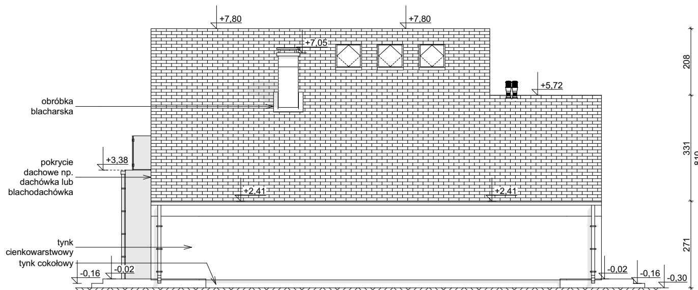
ELEWACJA BOCZNA
