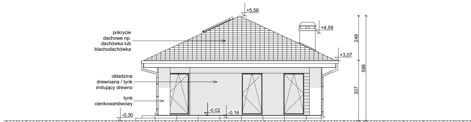
ELEWACJA OGRODOWA
