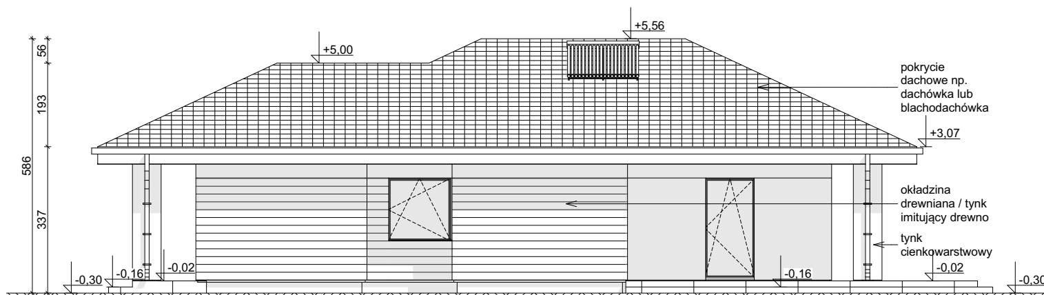
ELEWACJA BOCZNA
