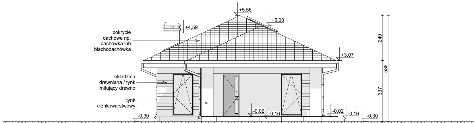
ELEWACJA FRONTOWA
