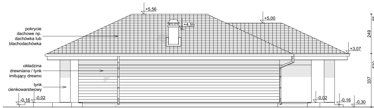
ELEWACJA BOCZNA
