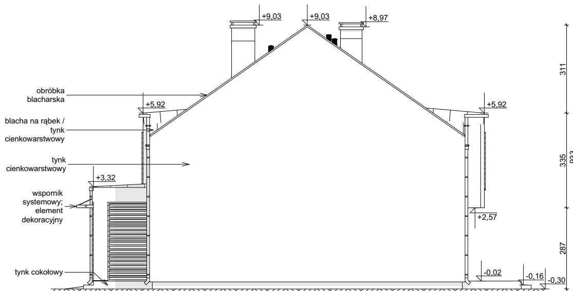
ELEWACJA BOCZNA
