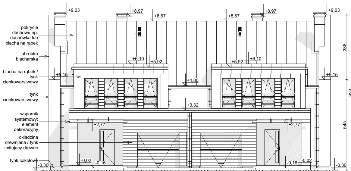
ELEWACJA FRONTOWA
