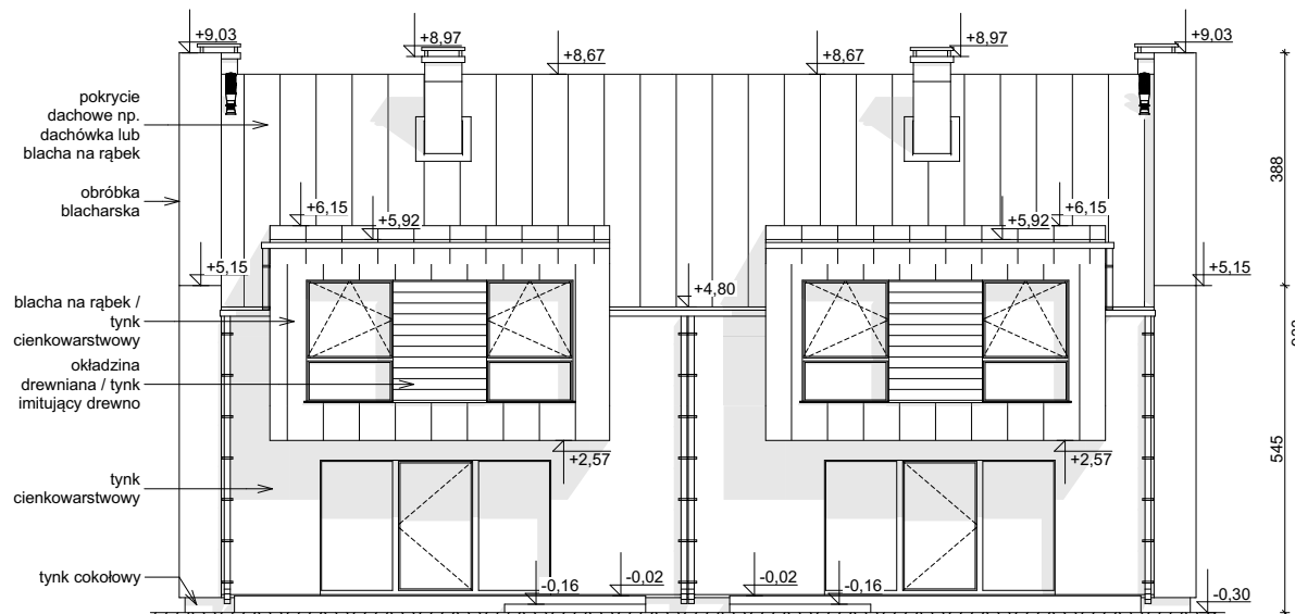
ELEWACJA OGRODOWA
