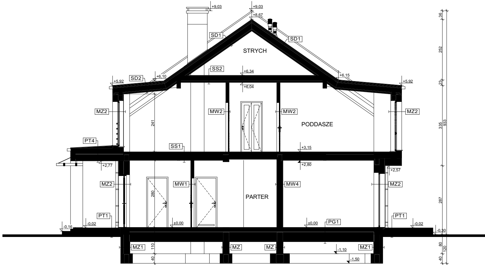
PRZEKRÓJ B-B
