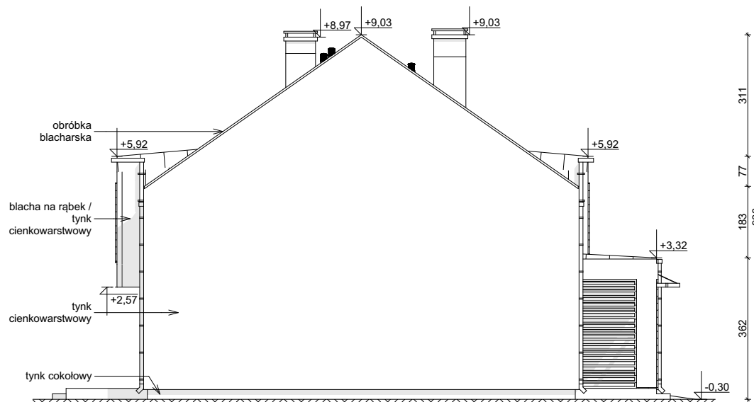
ELEWACJA BOCZNA
