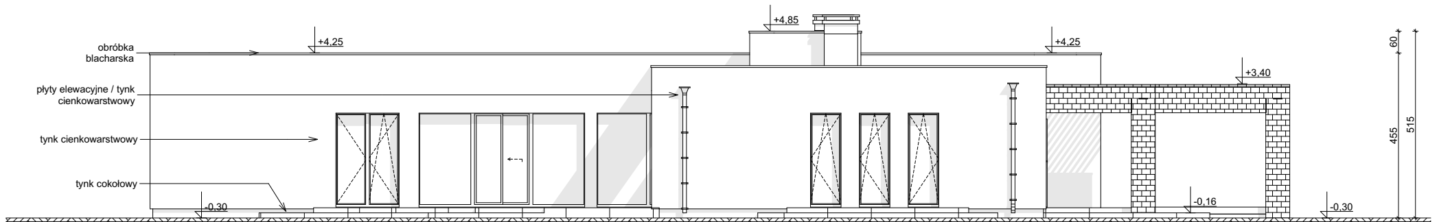
ELEWACJA BOCZNA
