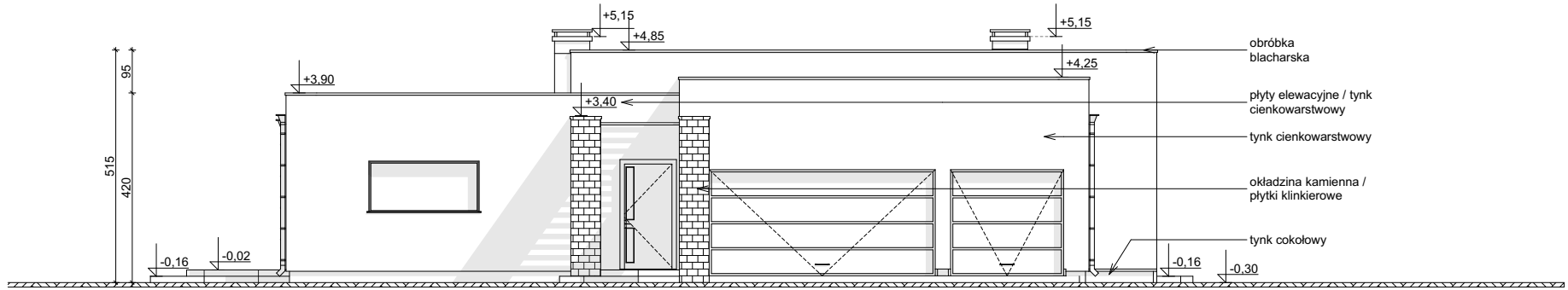
ELEWACJA FRONTOWA
